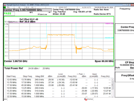
5G NR n77 25MHz BPSK High Channel RB64-0, ID:28498
