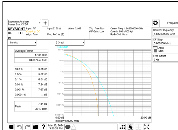
5G NR n25 35MHz BPSK Middle Channel, ID:50822
