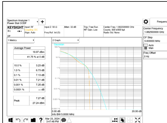
5G NR n25 20MHz BPSK Middle Channel, ID:50822
