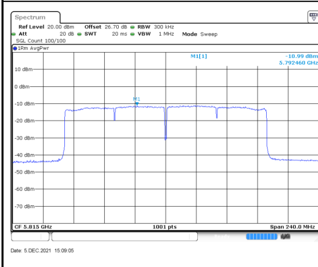
MIMO Ant. 4
