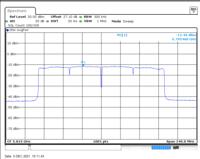
MIMO Ant. 3
