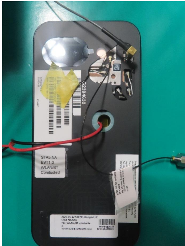
EUT
