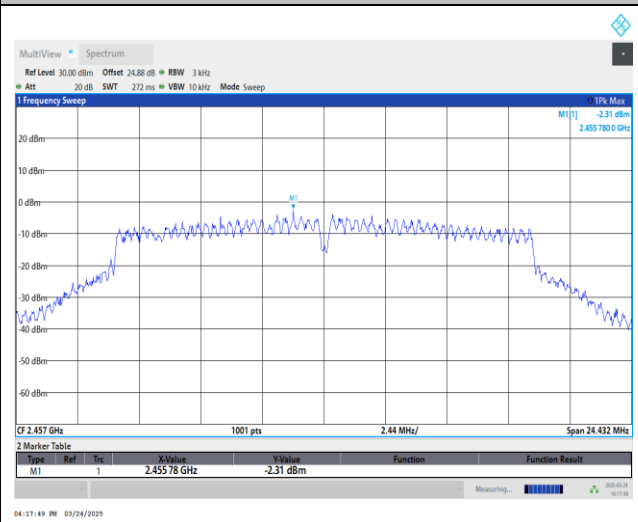
MIMO Ant 4
