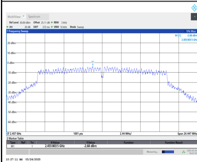
MIMO Ant 3
