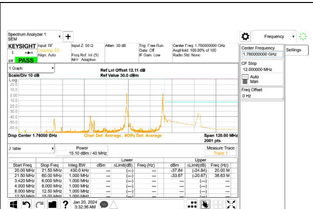
LTE B66C 20MHz + 20MHz QPSK High Ch RB1-99 + RB1-99
