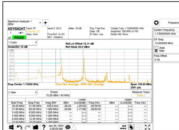
LTE B66C 20MHz + 20MHz QPSK Low Ch RB1-0 + RB1-0
