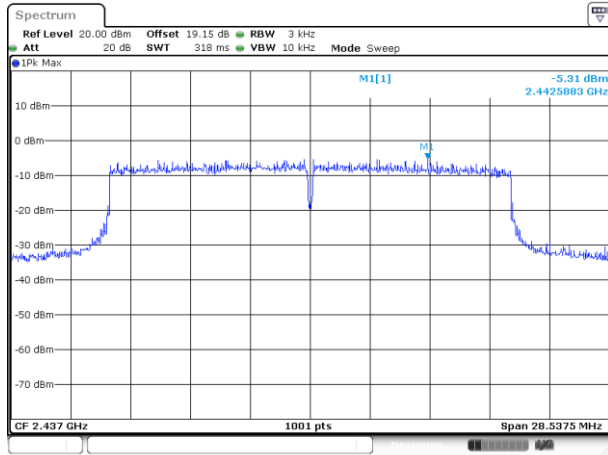
MIMO Ant. 4
