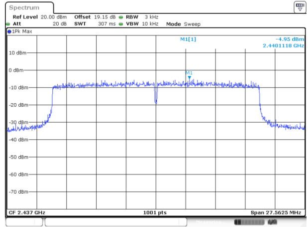
MIMO Ant. 3
