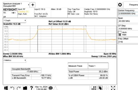
5G NR n41 20MHz BPSK Middle Channel RB50-0, ID:28498
