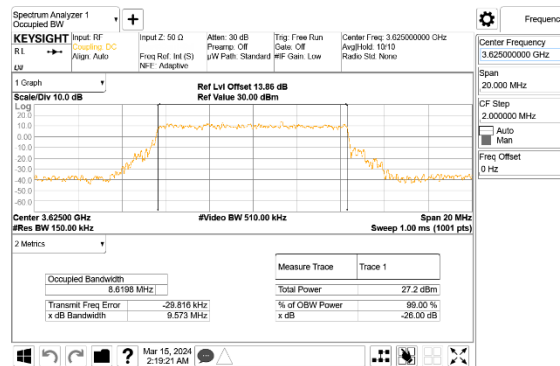
5G NR n48 10MHz BPSK Middle Channel RB24-0, ID:28498
