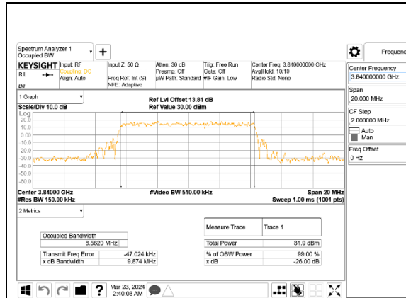
5G NR n77 10MHz BPSK Middle Channel RB24-0, ID:28498
