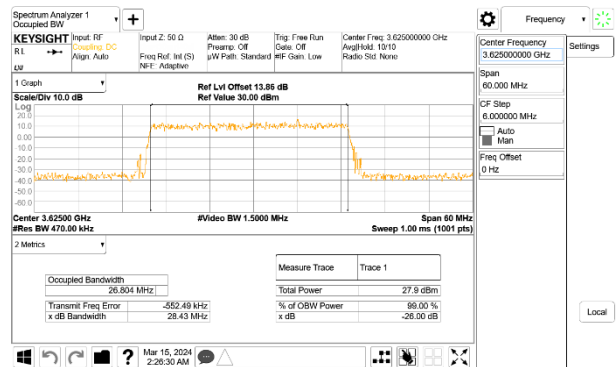
5G NR n48 30MHz BPSK Middle Channel RB75-0, ID:28498
