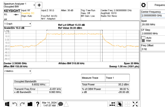
5G NR n41 10MHz BPSK Middle Channel RB24-0, ID:28498
