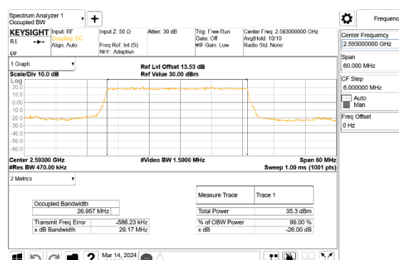
5G NR n41 30MHz BPSK Middle Channel RB75-0, ID:28498
