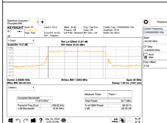
5G NR n77 20MHz BPSK Middle Channel RB50-0, ID:28498
