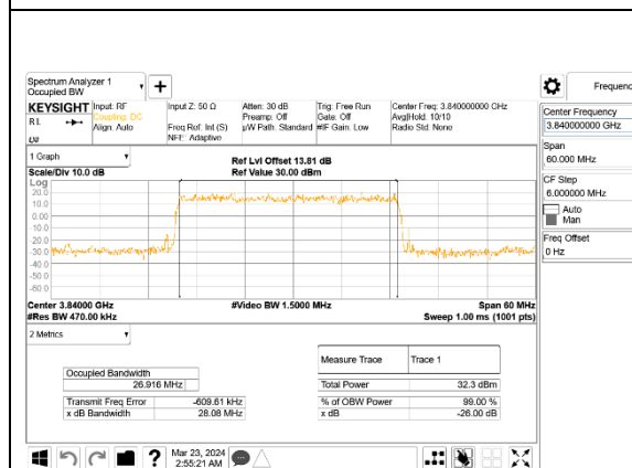
5G NR n77 30MHz BPSK Middle Channel RB75-0, ID:28498
