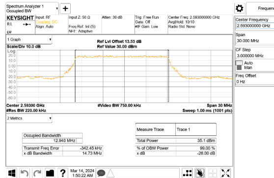
5G NR n41 15MHz BPSK Middle Channel RB36-0, ID:28498
