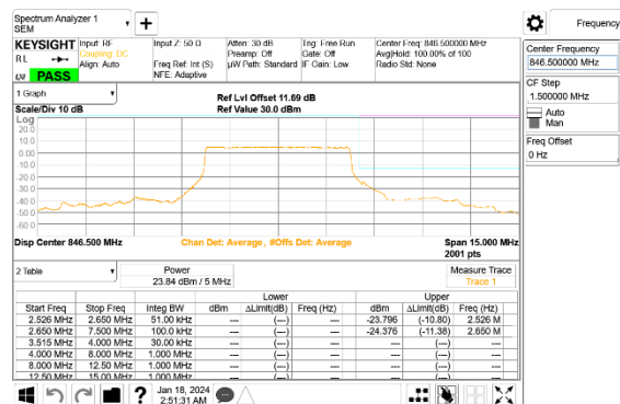
5G NR n5 5MHz BPSK High Channel RB25-0,ID:24898
