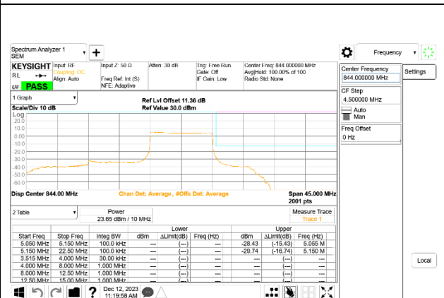
LTE B5 10MHz QPSK High Channel RB50-0, ID:32061
