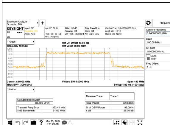
5G NR n77 90MHz BPSK Middle Channel RB243-0, ID:28498
