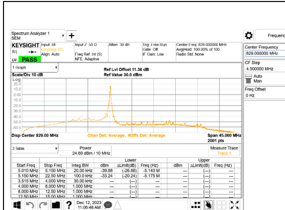
LTE B5 10MHz QPSK Low Channel RB1-0, ID:32061
