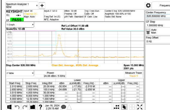
5G NR n5 5MHz BPSK Low Channel RB1-0,ID:24898
