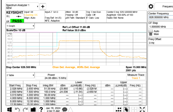
5G NR n5 5MHz BPSK Low Channel RB25-0,ID:24898
