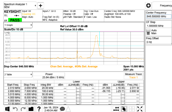
5G NR n5 5MHz BPSK High Channel RB1-24,ID:24898
