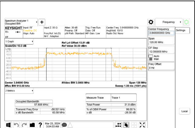
5G NR n77 60MHz BPSK Middle Channel RB162-0, ID:28498
