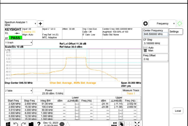
LTE B5 5MHz QPSK High Channel RB25-0, ID:32061
