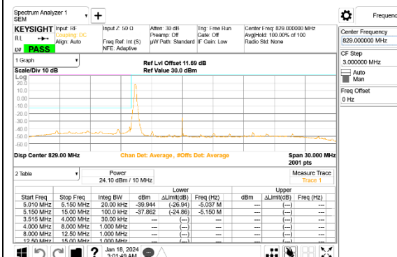
5G NR n5 10MHz BPSK Low Channel RB1-0,ID:24898
