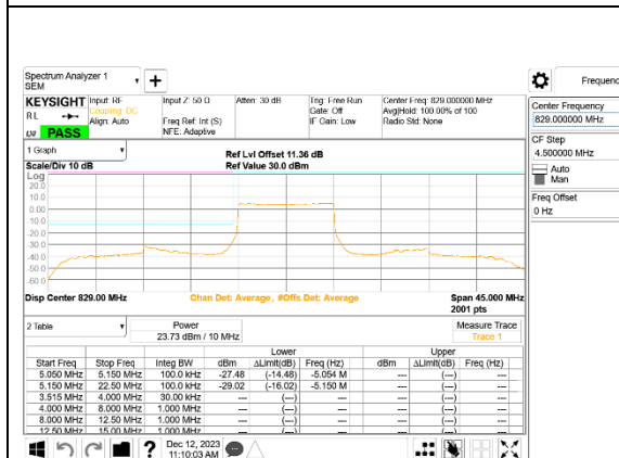
LTE B5 10MHz QPSK Low Channel RB50-0, ID:32061
