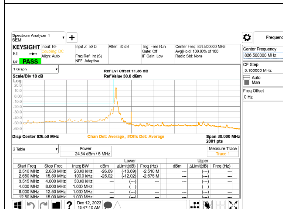
LTE B5 5MHz QPSK Low Channel RB1-0, ID:32061
