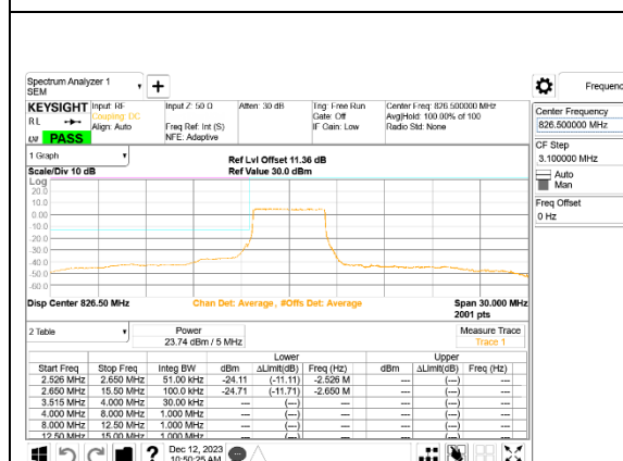
LTE B5 5MHz QPSK Low Channel RB25-0, ID:32061
