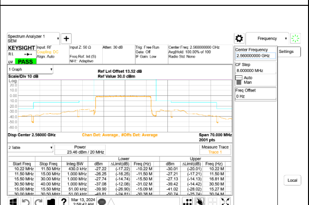
5G NR n7 20MHz BPSK High Channel RB100-0, ID:28498
