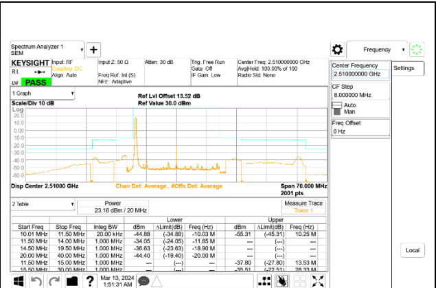
5G NR n7 20MHz BPSK Low Channel RB1-0, ID:28498
