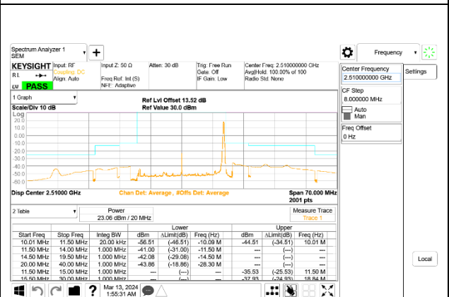
5G NR n7 20MHz BPSK Low Channel RB1-105, ID:28498
