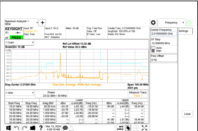
5G NR n7 30MHz BPSK Low Channel RB1-0, ID:28498
