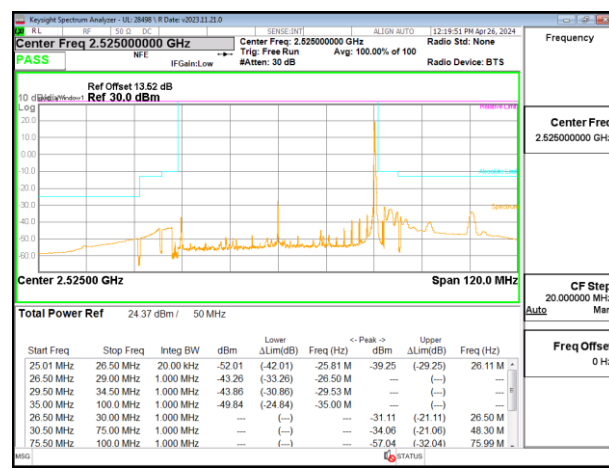
5G NR n7 50MHz BPSK Low Channel RB1-269, ID:28498
