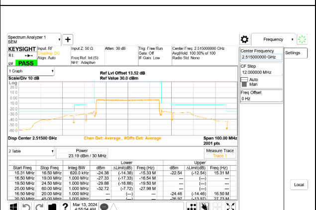
5G NR n7 30MHz BPSK Low Channel RB160-0, ID:28498
