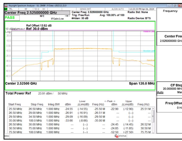
5G NR n7 50MHz BPSK Low Channel RB270-0, ID:28498
