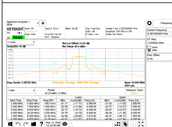
5G NR n7 5MHz BPSK High Channel RB25-0, ID:28498
