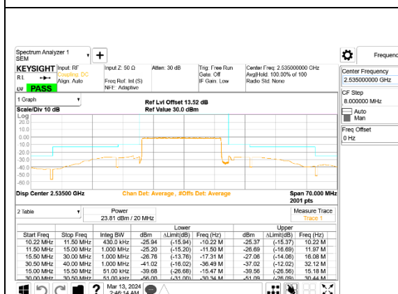
5G NR n7 20MHz BPSK Middle Channel RB100-0, ID:28498
