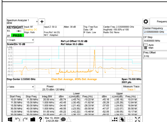
5G NR n7 20MHz BPSK Middle Channel RB1-105, ID:28498
