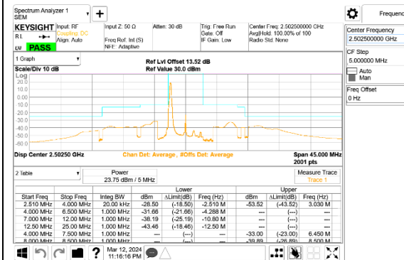
5G NR n7 5MHz BPSK Low Channel RB1-0, ID:28498
