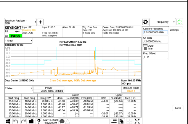
5G NR n7 30MHz BPSK Low Channel RB1-159, ID:28498
