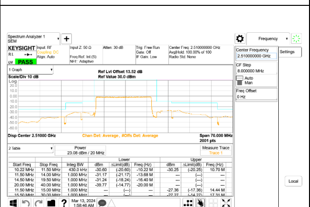
5G NR n7 20MHz BPSK Low Channel RB100-0, ID:28498
