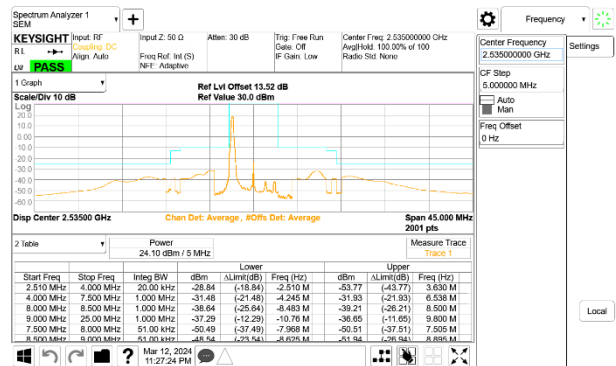
5G NR n7 5MHz BPSK Middle Channel RB1-0, ID:28498
