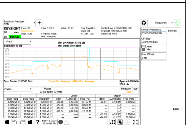
5G NR n7 10MHz BPSK Low Channel RB50-0, ID:28498
