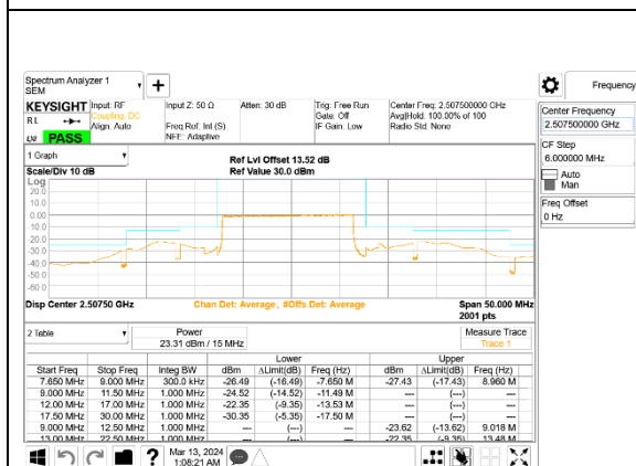
5G NR n7 15MHz BPSK Low Channel RB75-0, ID:28498
