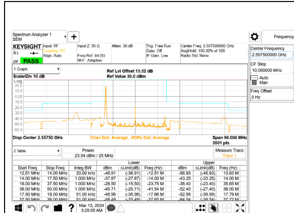
5G NR n7 25MHz BPSK High Channel RB1-0, ID:28498
