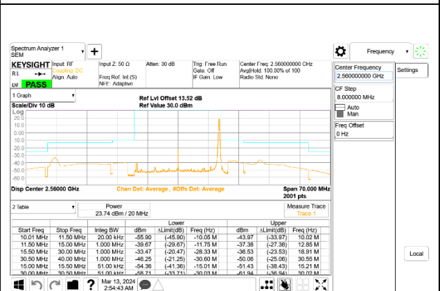
5G NR n7 20MHz BPSK High Channel RB1-105, ID:28498
