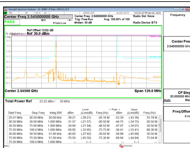
5G NR n7 50MHz BPSK High Channel RB1-0, ID:28498
