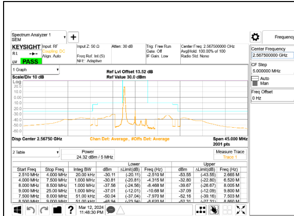
5G NR n7 5MHz BPSK High Channel RB1-0, ID:28498
