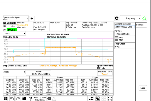
5G NR n7 30MHz BPSK High Channel RB160-0, ID:28498
