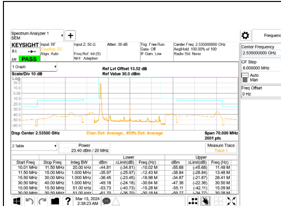
5G NR n7 20MHz BPSK Middle Channel RB1-0, ID:28498
