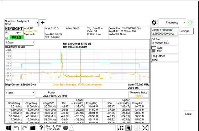
5G NR n7 20MHz BPSK High Channel RB1-0, ID:28498
