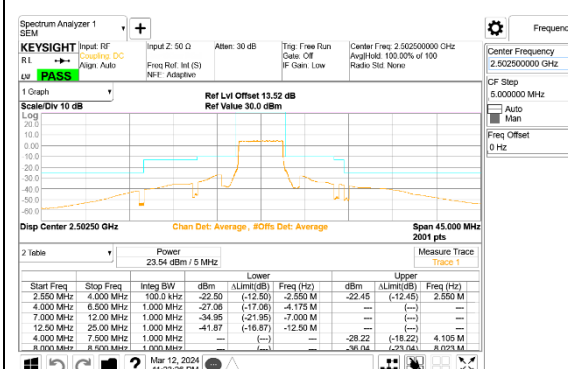
5G NR n7 5MHz BPSK Low Channel RB25-0, ID:28498
