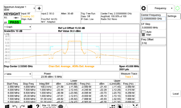
5G NR n7 5MHz BPSK Middle Channel RB25-0, ID:28498
