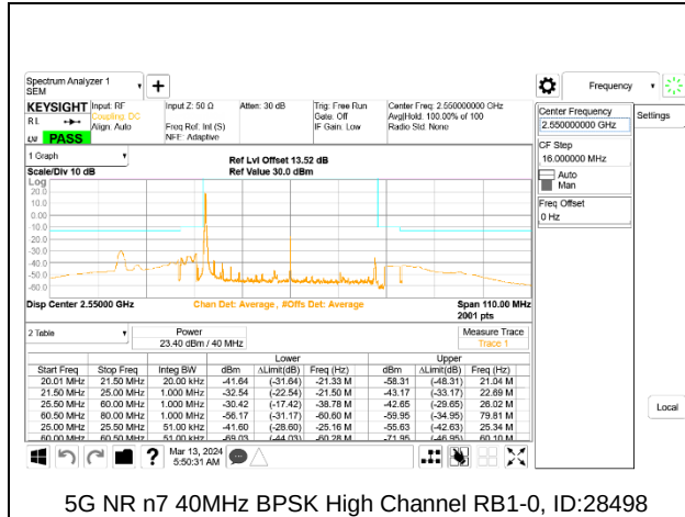
5G NR n7 40MHz BPSK High Channel RB1-0, ID:28498
