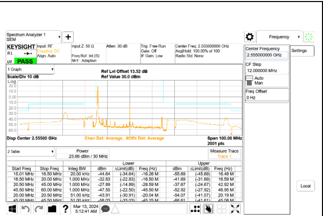
5G NR n7 30MHz BPSK High Channel RB1-0, ID:28498
