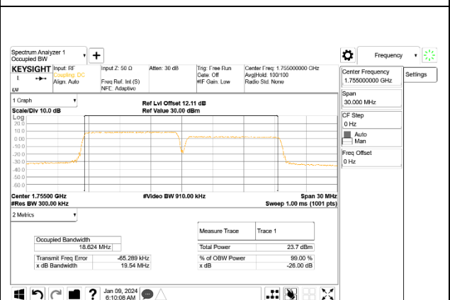
LTE B66B 10MHz + 10MHz QPSK RB50-0 + RB50-0 ID:32061
