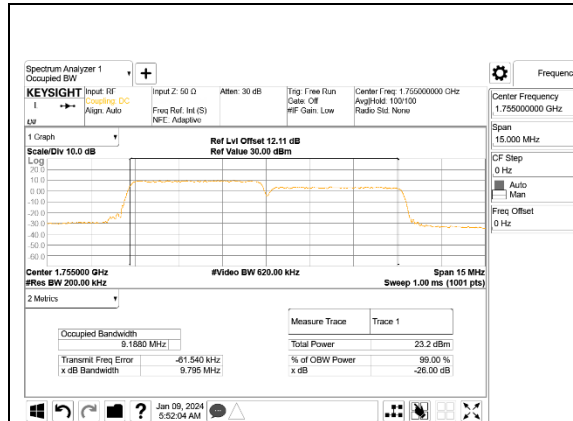
LTE B66B 5MHz + 5MHz QPSK RB25-0 + RB25-0 ID:32061
