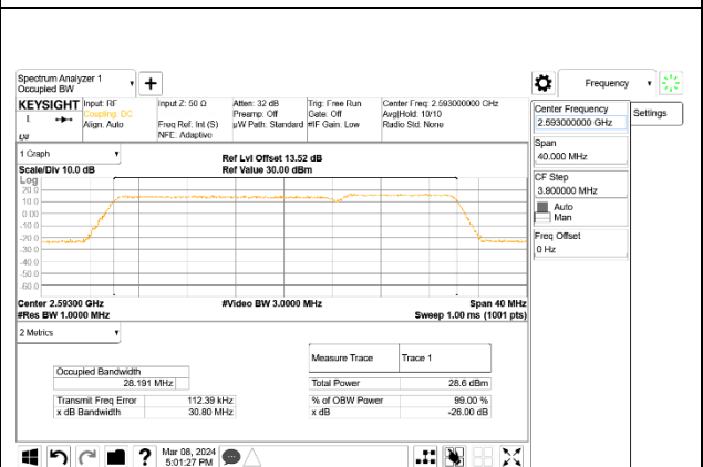
LTE B41 20MHz + 10MHz QPSK RB100-0 + RB50-0 ID:32061
