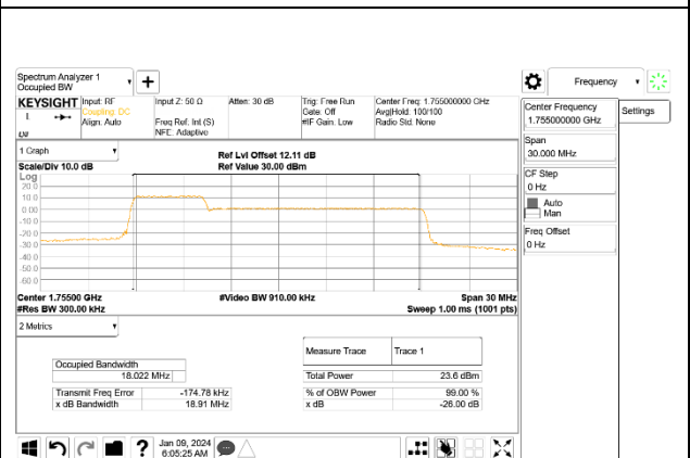
LTE B66B 5MHz + 15MHz QPSK RB25-0 + RB75-0 ID:32061
