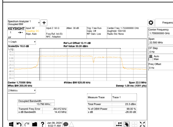
LTE B66B 10MHz + 5MHz QPSK RB50-0 + RB25-0 ID:32061
