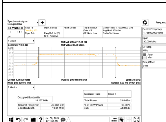
LTE B66B 15MHz + 5MHz QPSK RB75-0 + RB25-0 ID:32061
