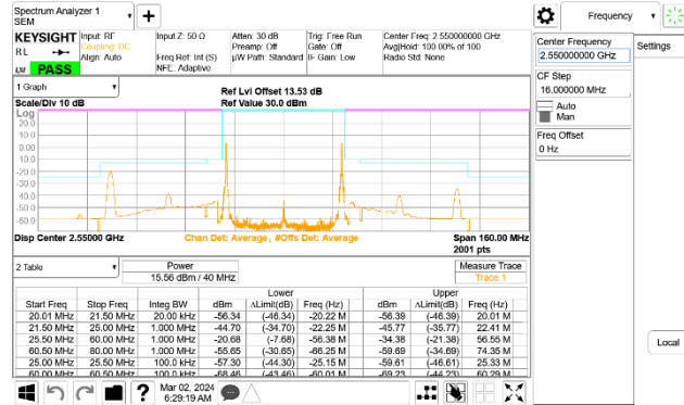
LTE B7 20MHz + 20MHz 16QAM High Ch RB1-0 + RB1-99 ID:32061
