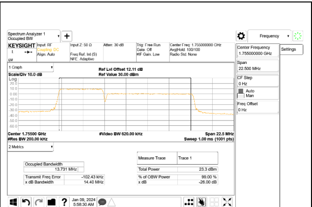
LTE B66B 5MHz + 10MHz QPSK RB25-0 + RB50-0 ID:32061
