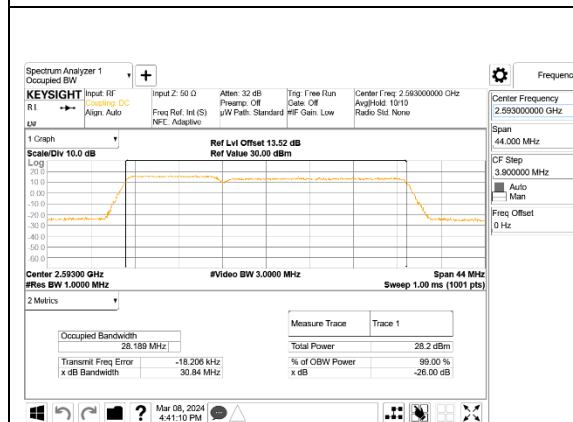
LTE B41 10MHz + 20MHz QPSK RB50-0 + RB100-0 ID:32061
