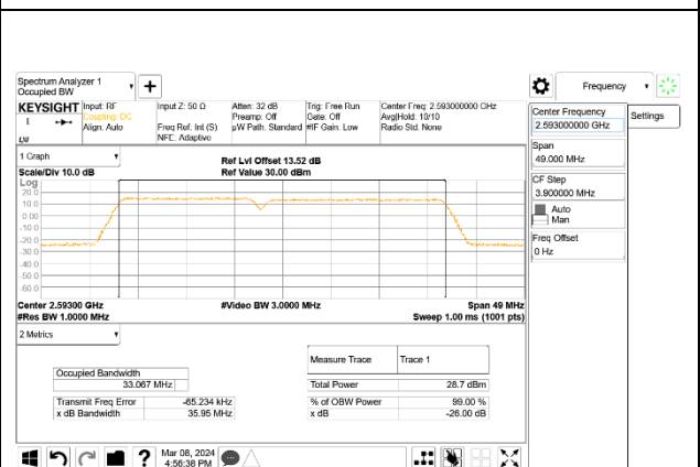
LTE B41 15MHz + 20MHz QPSK RB75-0 + RB100-0 ID:32061
