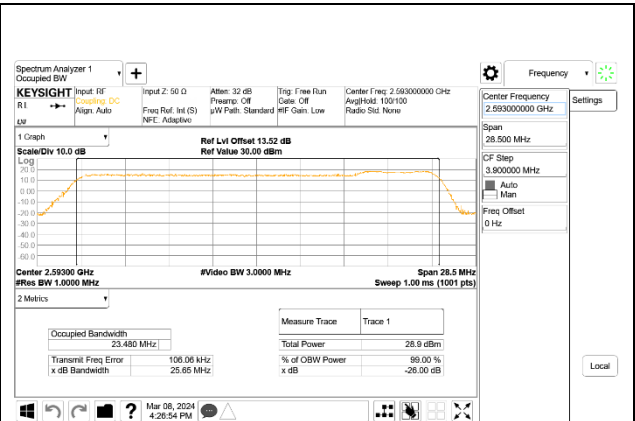
LTE B41 20MHz + 5MHz QPSK RB100-0 + RB25-0 ID:32061
