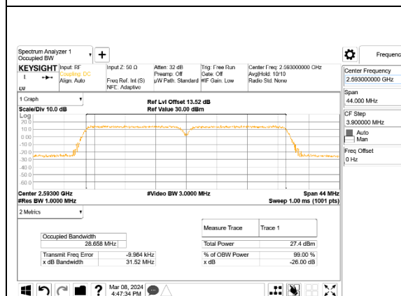
LTE B41 15MHz + 15MHz QPSK RB75-0 + RB75-0 ID:32061
