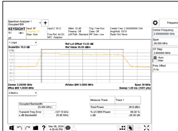
LTE B41 5MHz + 20MHz QPSK RB25-0 + RB100-0 ID:32061
