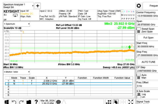
LTE B7 20MHz + 20MHz QPSK Middle Ch RB1-99 + RB1-0 ID:32061
