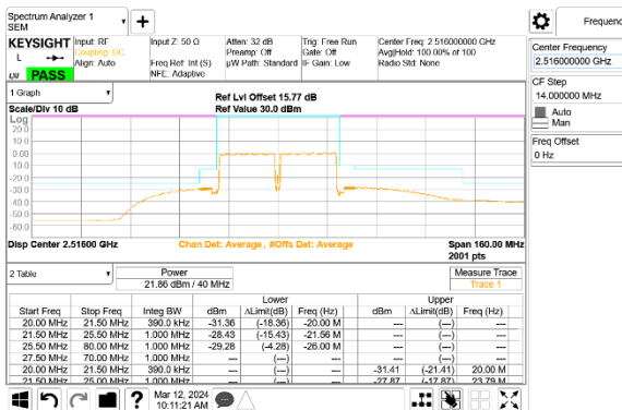
LTE B41 20MHz + 20MHz QPSK Low Ch RB100-0 + RB100-0 ID:32061
