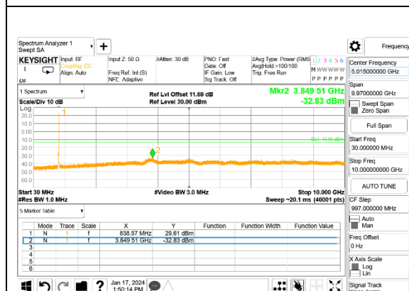
LTE B5 10MHz + 10MHz QPSK High Ch RB1-49 + RB1-0 ID:32061
