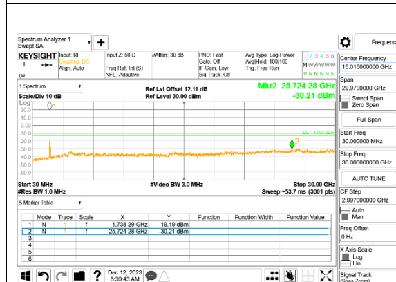
LTE B66C 20MHz + 20MHz QPSK High Ch RB1-99 + RB1-0 ID:32061
