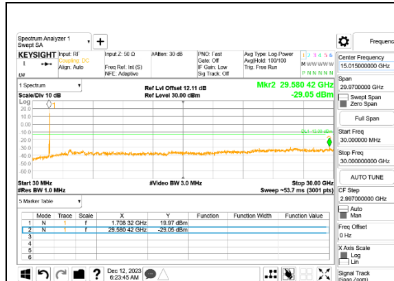
LTE B66C 20MHz + 20MHz QPSK Low Ch RB1-99 + RB1-0 ID:32061
