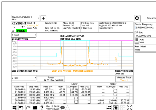
LTE B41 20MHz + 20MHz QPSK Low Ch RB1-0 + RB1-99 ID:32061
