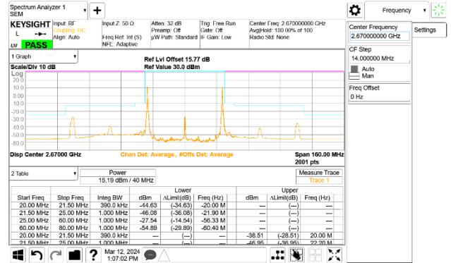
LTE B41 20MHz + 20MHz 16QAM High Ch RB1-0 + RB1-99 ID:32061
