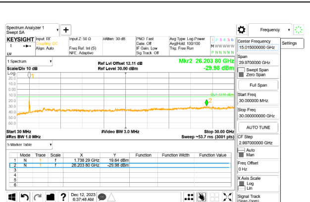
LTE B66C 20MHz + 20MHz QPSK Middle Ch RB1-99 + RB1-0 ID:32061
