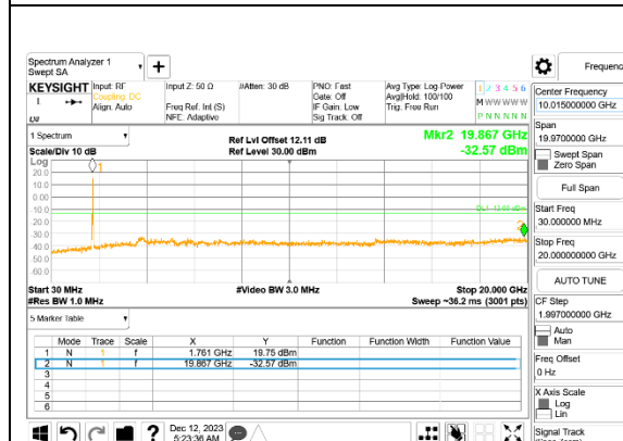
LTE B66B 10MHz + 10MHz QPSK High Ch RB1-49 + RB1-0 ID:32061
