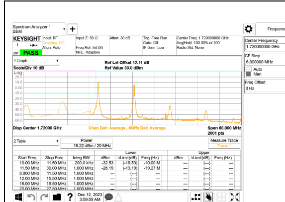
LTE B66B 10MHz + 10MHz QPSK Low Ch RB1-0 + RB1-0 ID:32061
