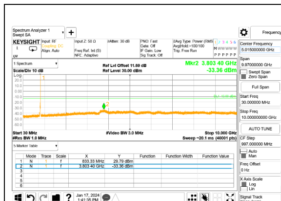
LTE B5 10MHz + 10MHz QPSK Low Ch RB1-49 + RB1-0 ID:32061
