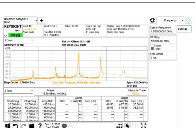
LTE B66C 20MHz + 20MHz 16QAM High Ch RB1-99 + RB1-99 ID:32061
