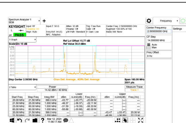
LTE B41 20MHz + 20MHz 16QAM Mid Ch RB1-0 + RB1-99 ID:32061
