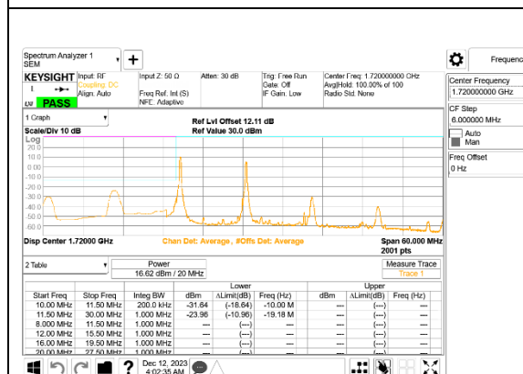
LTE B66B 10MHz + 10MHz 16QAM Low Ch RB1-0 + RB1-0 ID:32061
