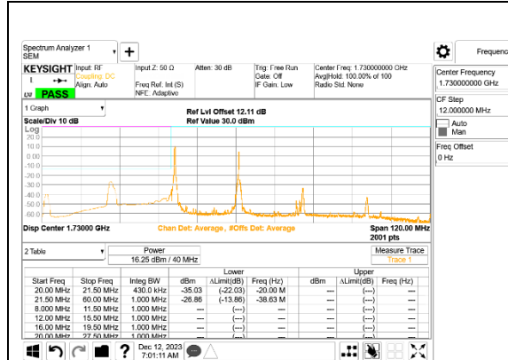
LTE B66C 20MHz + 20MHz QPSK Low Ch RB1-0 + RB1-0 ID:32061
