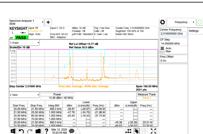
LTE B41 20MHz + 20MHz 16QAM Low Ch RB1-0 + RB1-99 ID:32061
