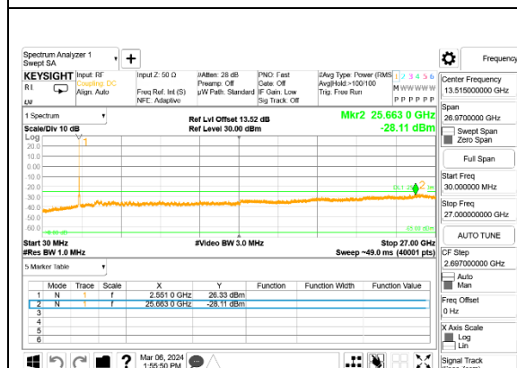
LTE B7 20MHz + 20MHz QPSK High Ch RB1-99 + RB1-0 ID:32061
