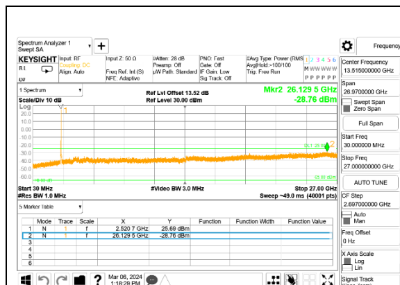
LTE B7 20MHz + 20MHz QPSK Low Ch RB1-99 + RB1-0 ID:32061
