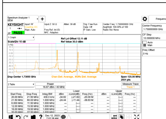
LTE B66C 20MHz + 20MHz 16QAM Low Ch RB1-0 + RB1-0 ID:32061
