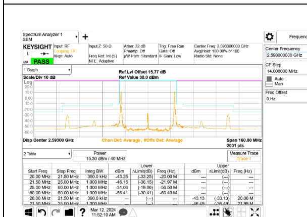
LTE B41 20MHz + 20MHz QPSK Mid Ch RB1-0 + RB1-99 ID:32061
