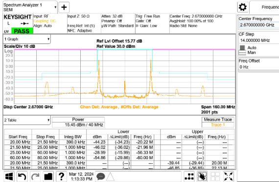
LTE B41 20MHz + 20MHz QPSK High Ch RB1-0 + RB1-99 ID:32061
