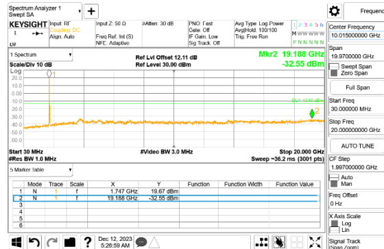
LTE B66B 10MHz + 10MHz QPSK Middle Ch RB1-49 + RB1-0 ID:32061
