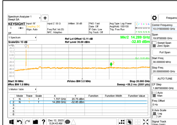
LTE B66B 10MHz + 10MHz QPSK Low Ch RB1-49 + RB1-0 ID:32061
