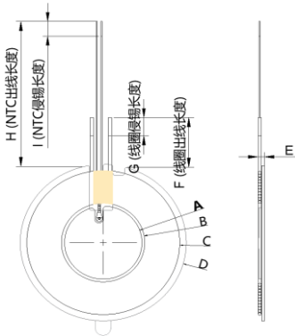
图纸
