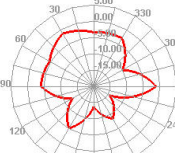
5490.000MHz E1
