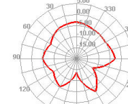
5490.000MHz E2
