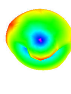
5850.000MHz E1
