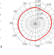
5850.000MHz E2
