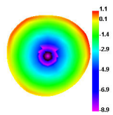
2450.000MHz E1
