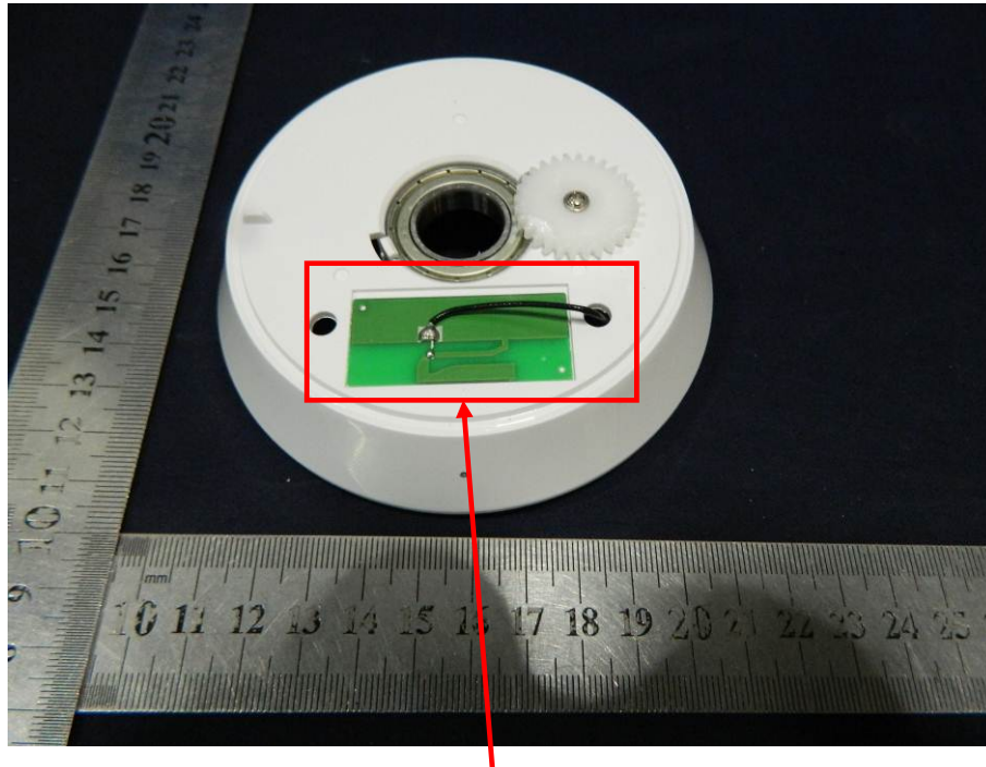
Antenna2
