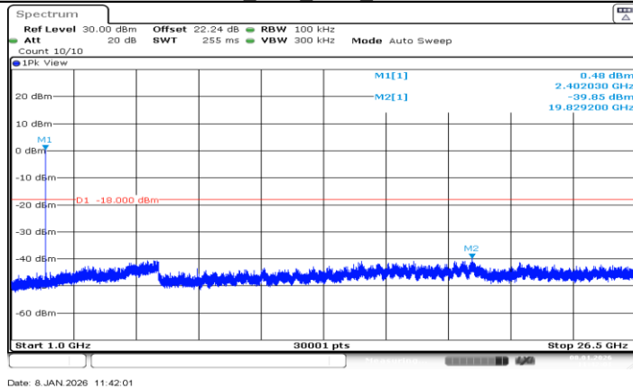
2DH5_Ant1_2402_1000~26500
