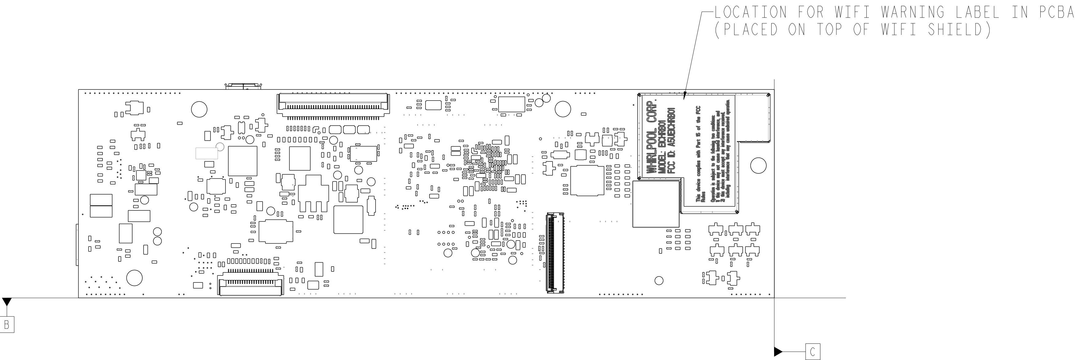
REBEL PCBA P/N W11324868 SCALE 2:1
