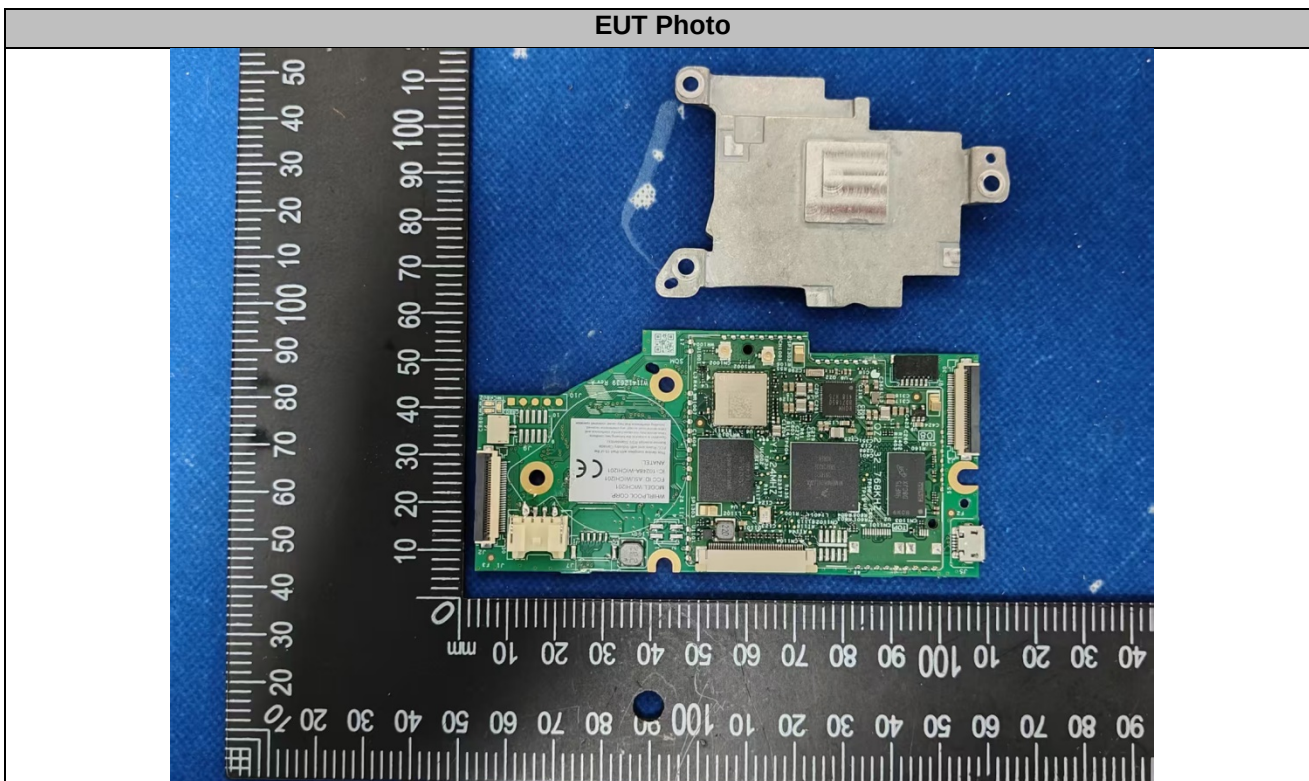
EUT Photo
