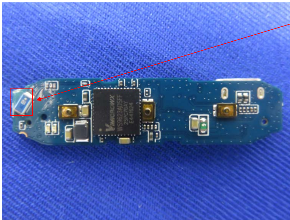
BT Anten
