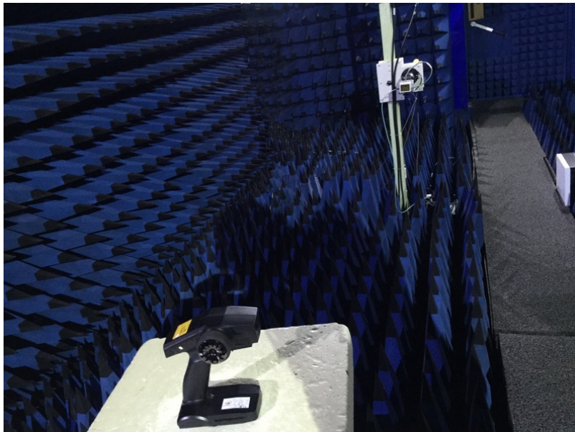
SE 18GHz-25GHz
