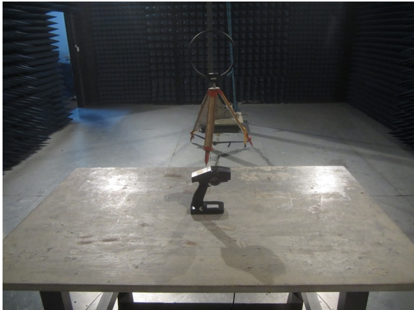
SE Below 30MHz
