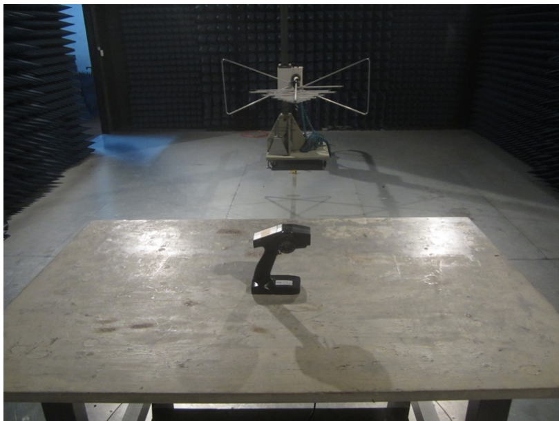
SE 30MHz-1GHz
