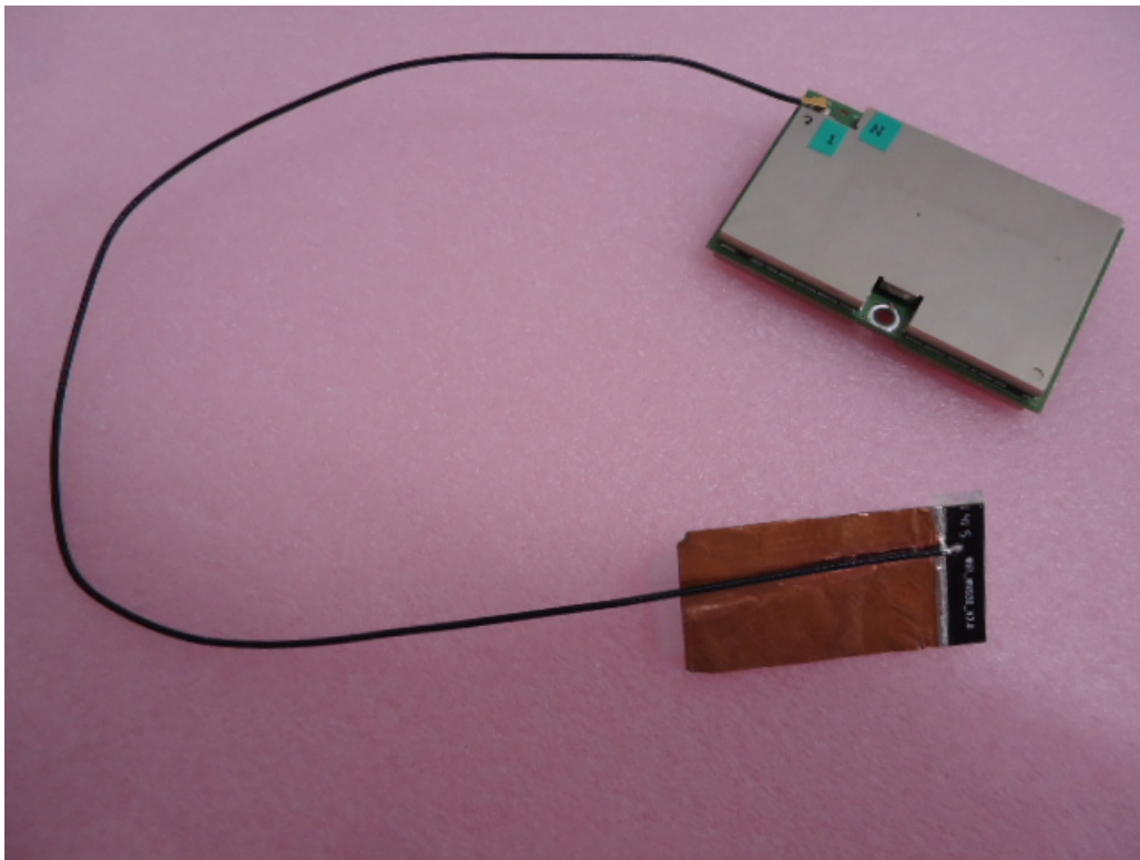
L08RF009-CS-R (PIFA) Whole
