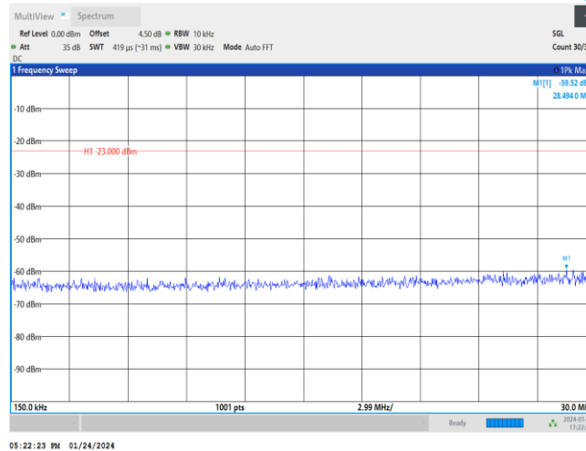
Band26-10MHz-QPSK-26740-1RB#0-Range2:0.15~30MHz
