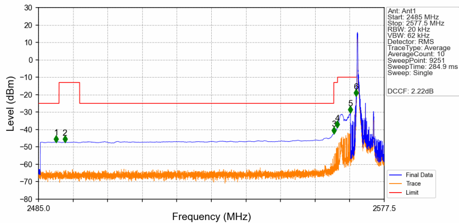
Band38_5MHz_QPSK_LCH_2572.5MHz_RB_1_0_NTNV
