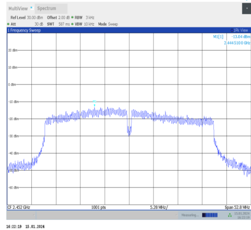
11n40ISO-Ant1-2452-PASS
