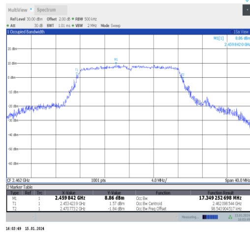
11g-Ant1-2462
