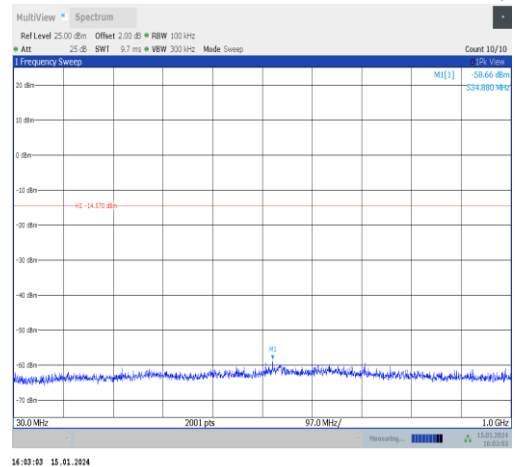
11g-Ant1-2437-30~1000-PASS
