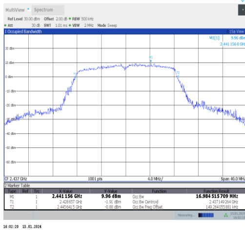
11g-Ant1-2437
