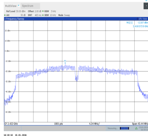
11n40ISO-Ant1-2422-PASS
