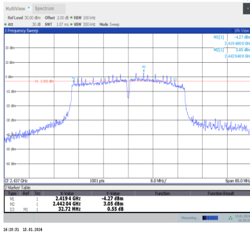
11n40ISO-Ant1-2437-PASS
