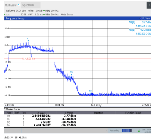
11n40ISO-Ant1-2452-PASS
