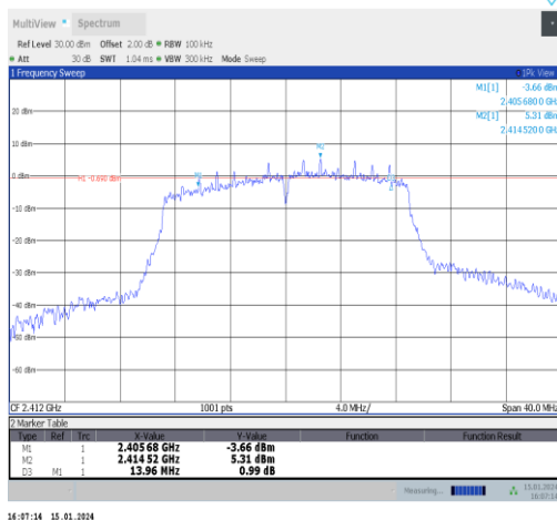
11n20ISO-Ant1-2412-PASS
