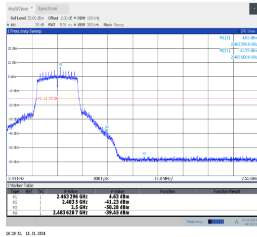
11n20ISO-Ant1-2462-PASS
