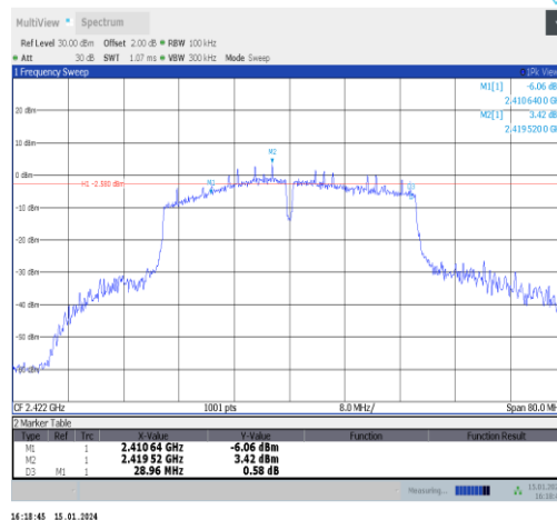
11n40ISO-Ant1-2422-PASS
