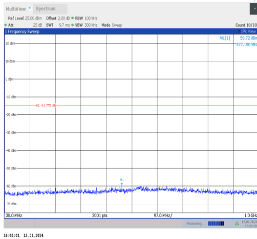
11g-Ant1-2412-30~1000-PASS
