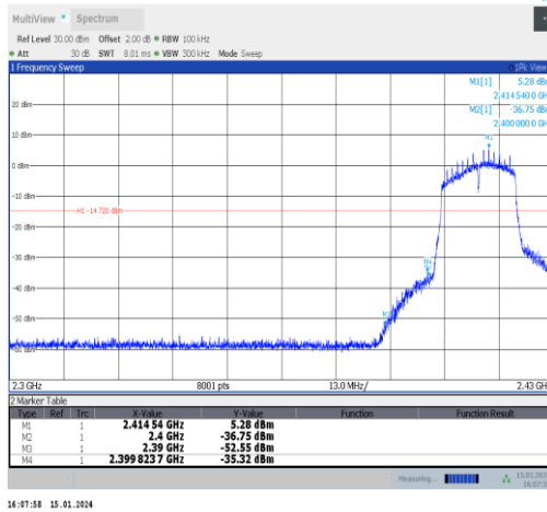
11n20ISO-Ant1-2412-PASS
