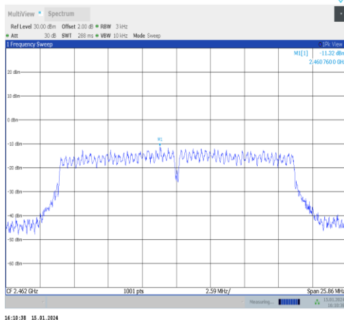
11n20ISO-Ant1-2462-PASS
