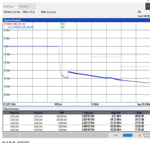
Band41_10MHz_QPSK_41190_50RB#0
