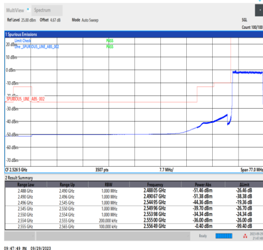
Band41_10MHz_QPSK_40290_50RB#0
