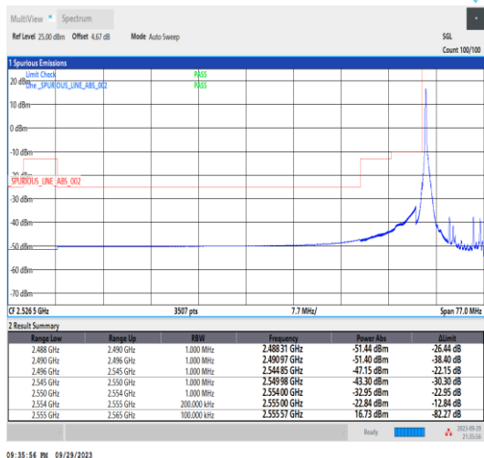
Band41_10MHz_QPSK_40290_1RB#0
