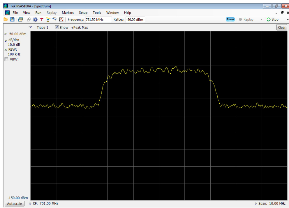
WCDMA Input_746-757 MHz
