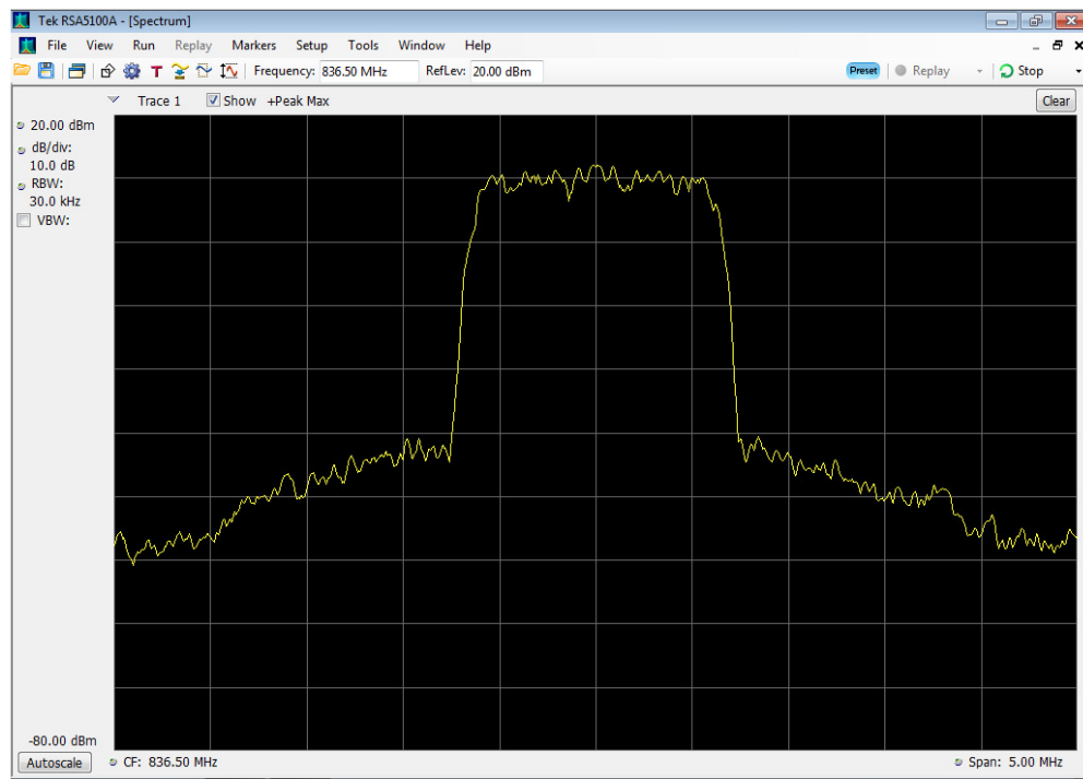
CDMA output_824-849MHz
