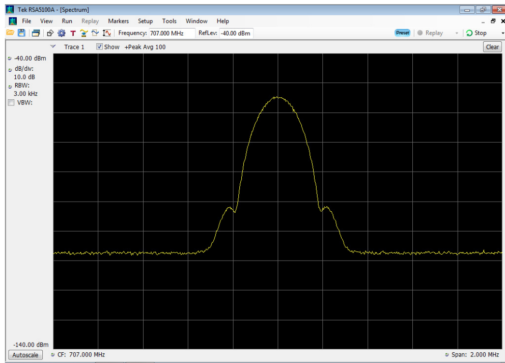
GSM Input_698 - 716 MHz
