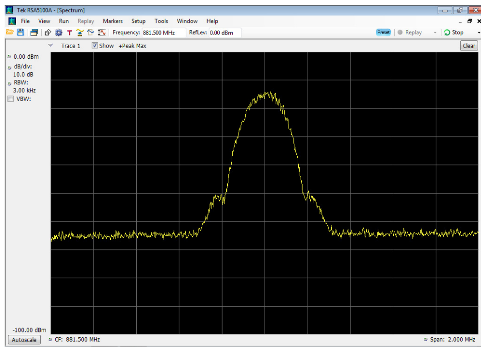
GSM output_869-894 MHz
