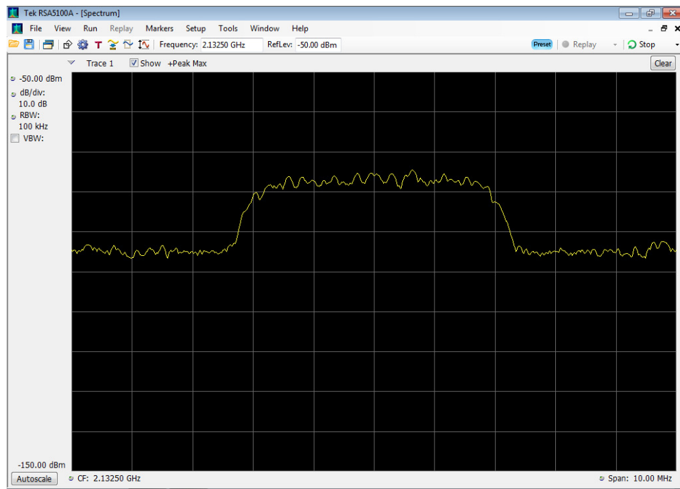
WCDMA Input_2110-2155 MHz
