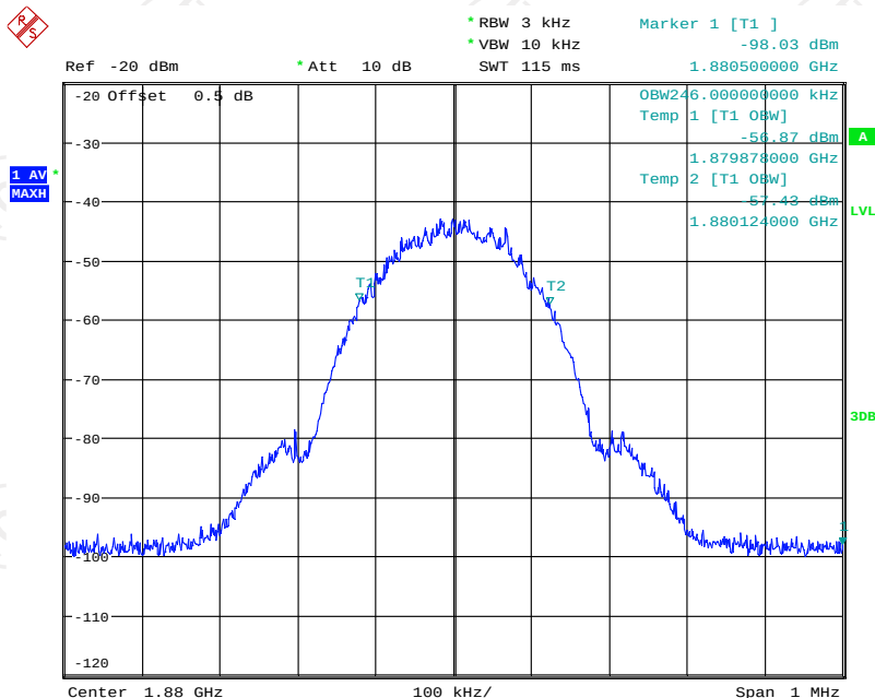
Band2 GSM UL Input
