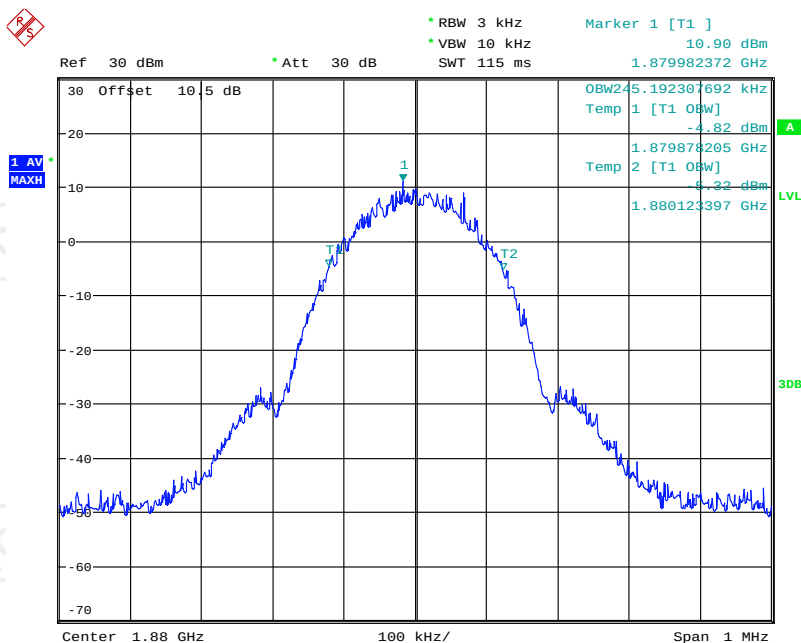
Band2 GSM UL output
