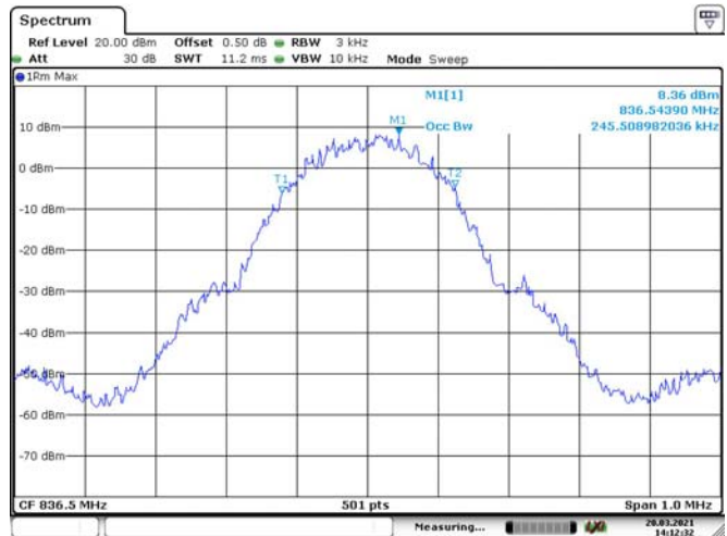
GSM-Output
