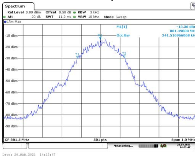
CDMA-Output
