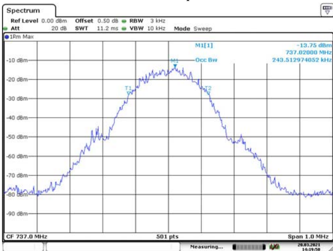
GSM-Output
