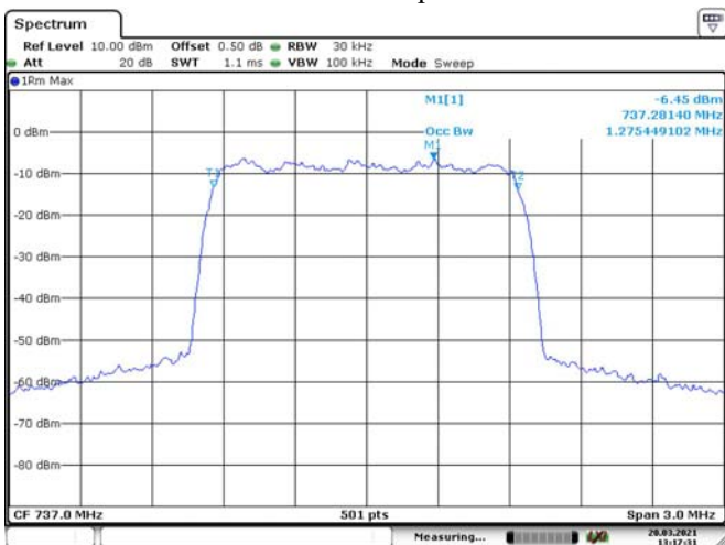
CDMA-Output
