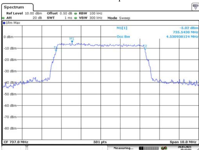
WCDMA-Output
