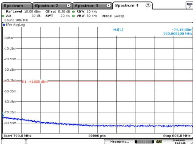
Upper 700M Band-5
