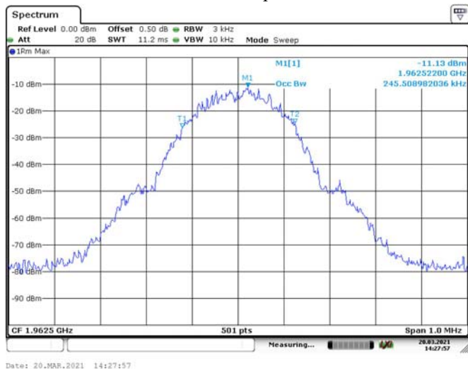
CDMA-Output
