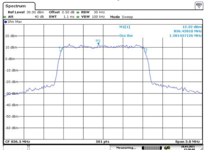
CDMA-Output
