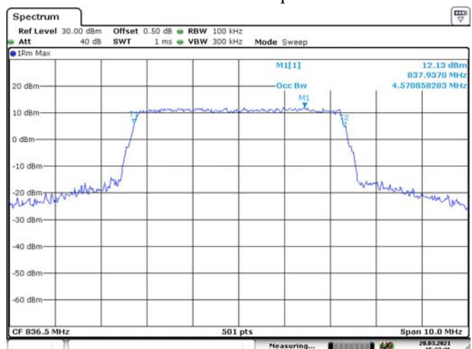
WCDMA-Output
