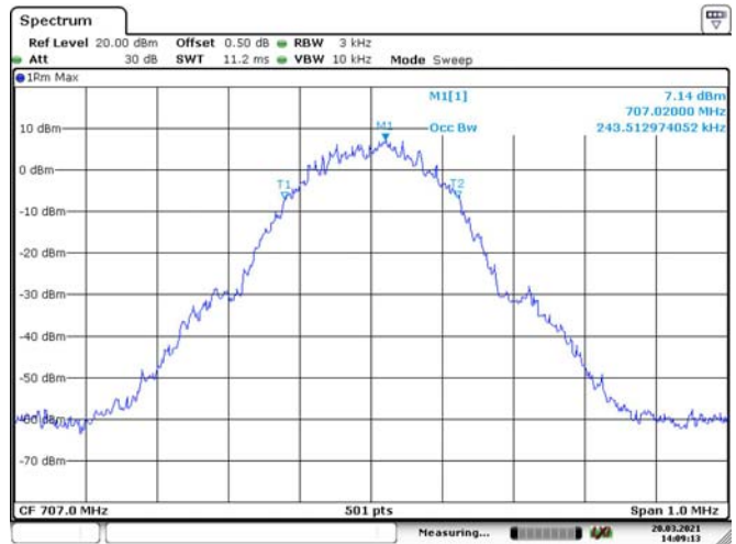
GSM-Output
