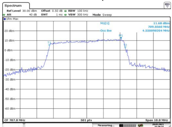
WCDMA-Output
