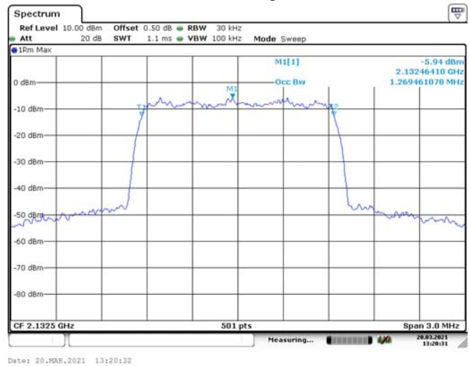
WCDMA-Output
