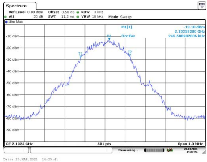
CDMA-Output
