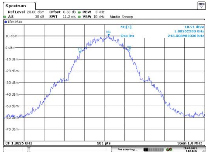
GSM-Output
