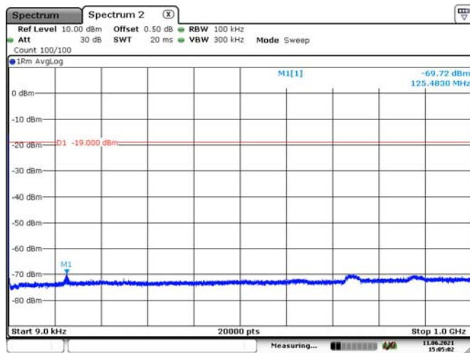
AWS Band-1
