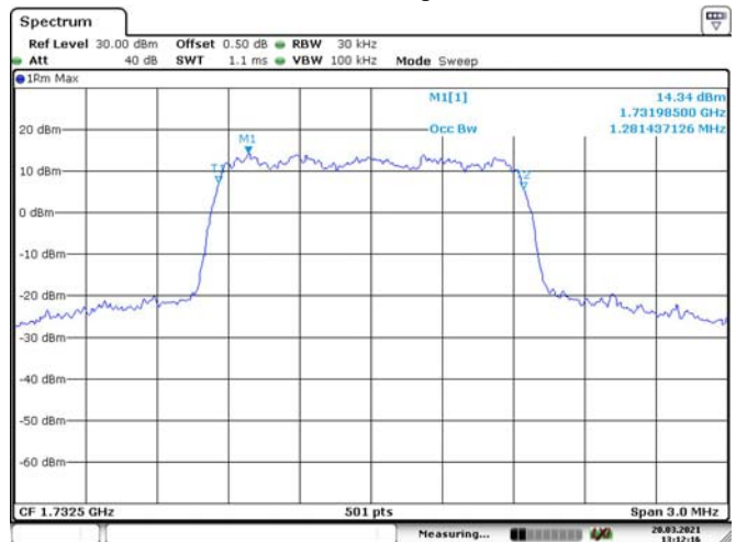
CDMA-Output
