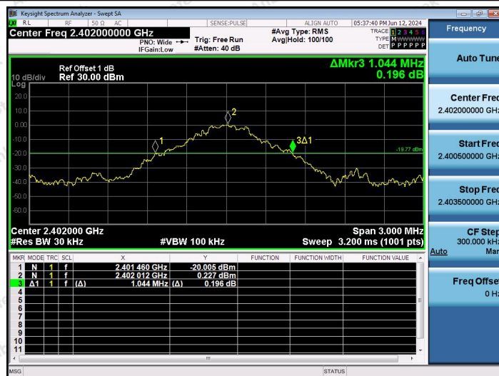
2.4G-Ant1-2402
