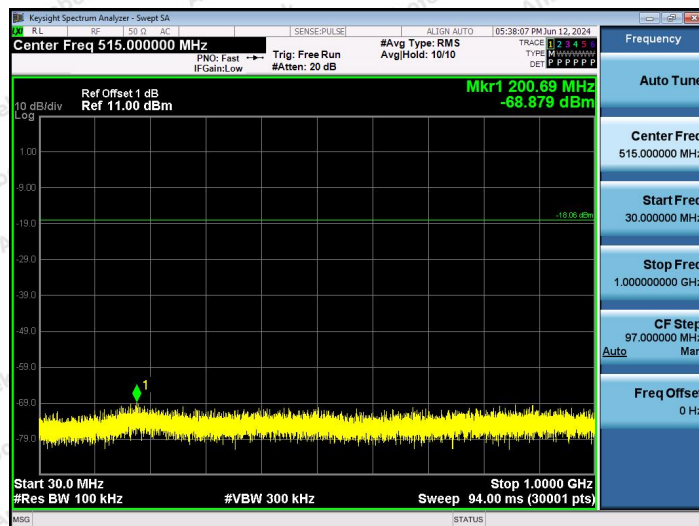
2.4G-Ant1-2402-30~1000-PASS
