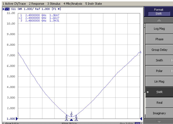
VSWR
