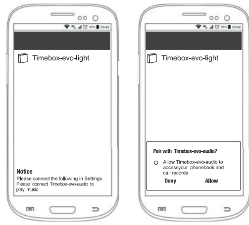
안드로이드 시스템
