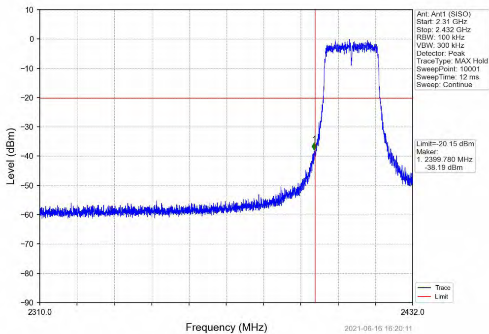
802.11n(HT20)_LCH_2412MHz_Ant1 (SISO)_NTNV
