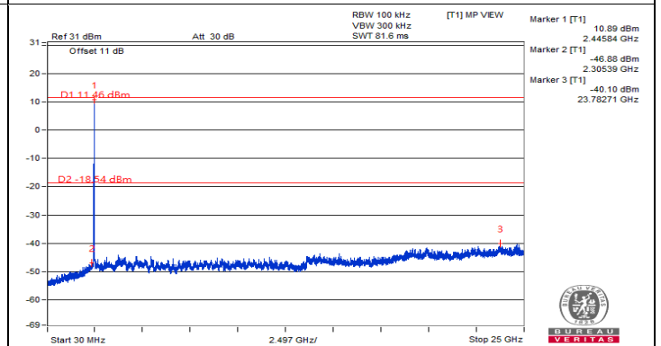
Chain 3 : CH 6
