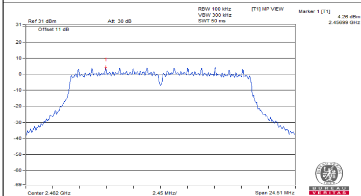
Chain 3 : CH 11
