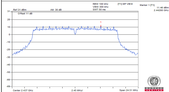
Chain 3 : CH 6
