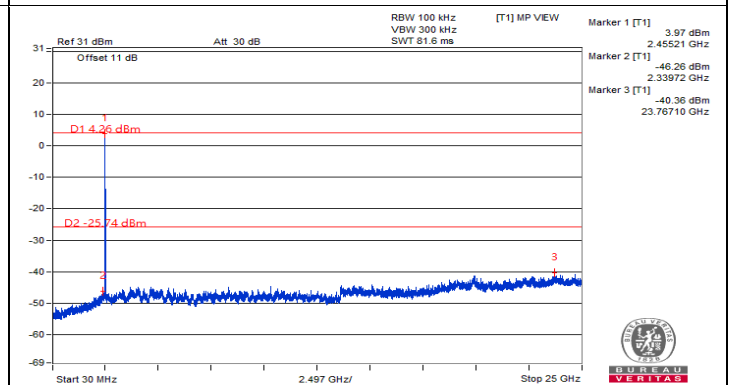
Chain 3 : CH 11
