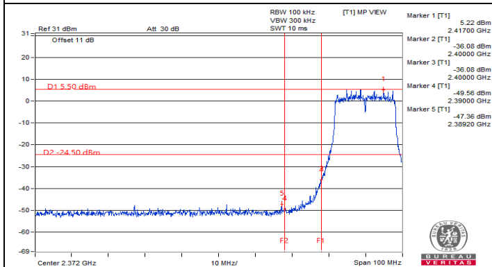
Chain 3 : CH 1 Band edge
