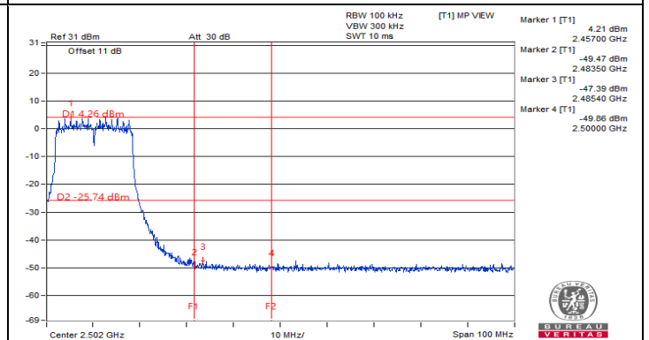
Chain 3 : CH 11 Band edge
