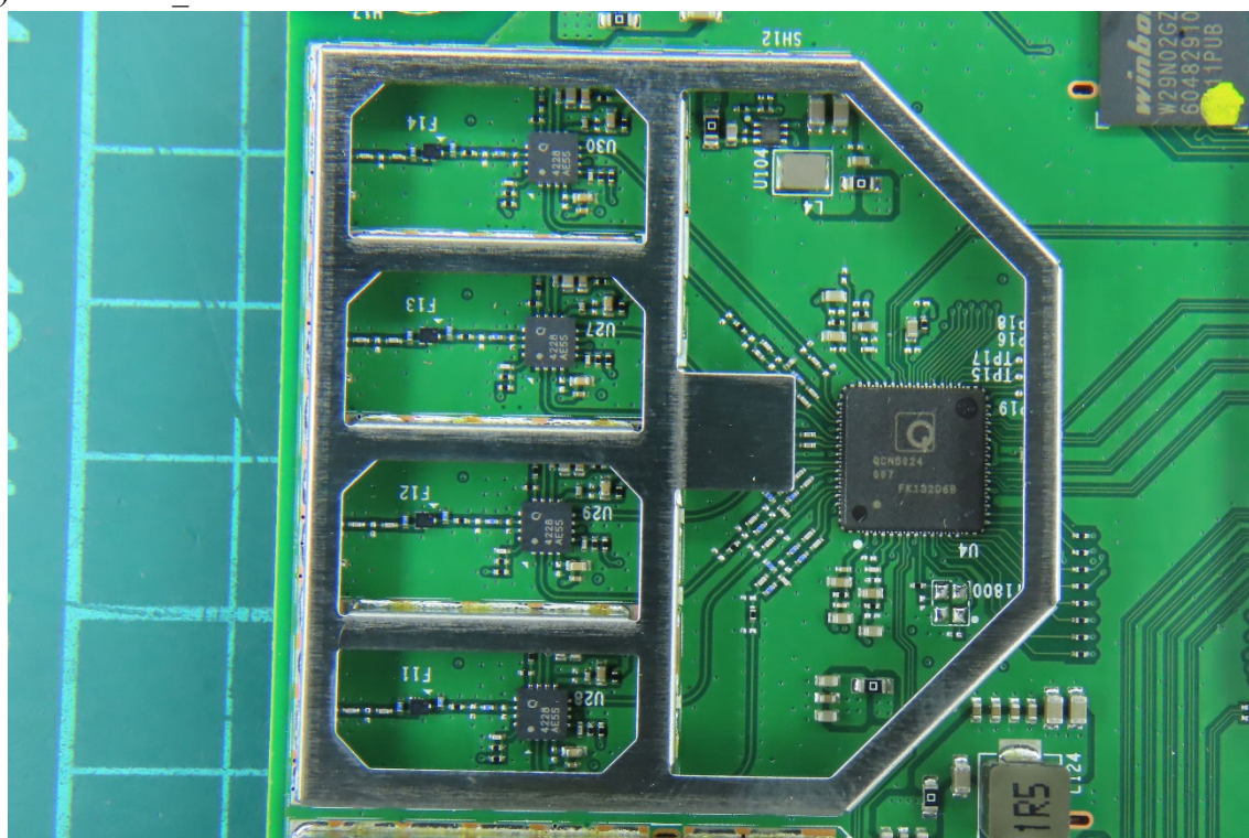
(10) EUT Photo_2.4GHz Module
