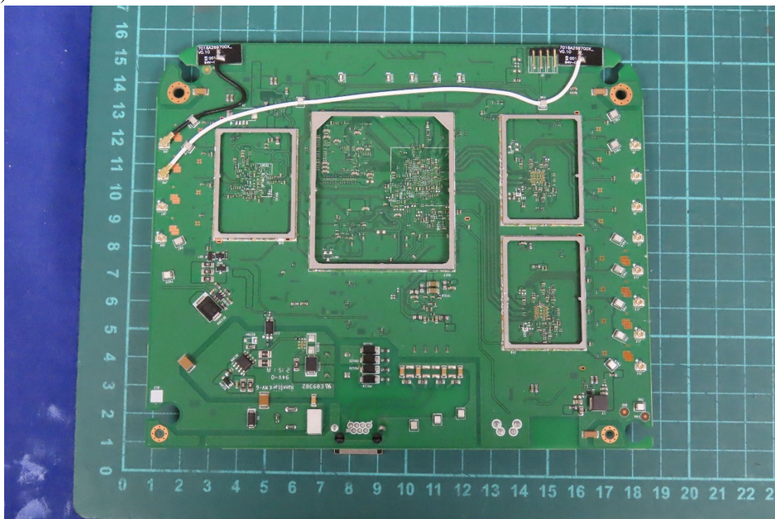
(6) EUT Photo
