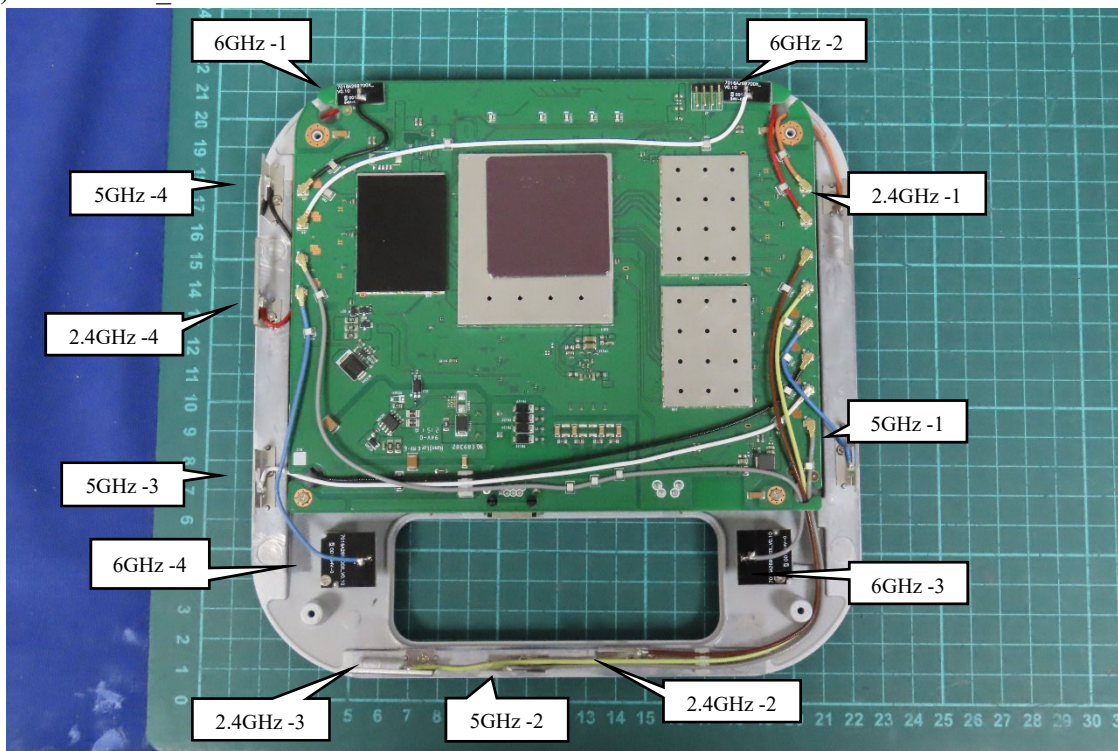
(2) EUT Photo_Antenna
