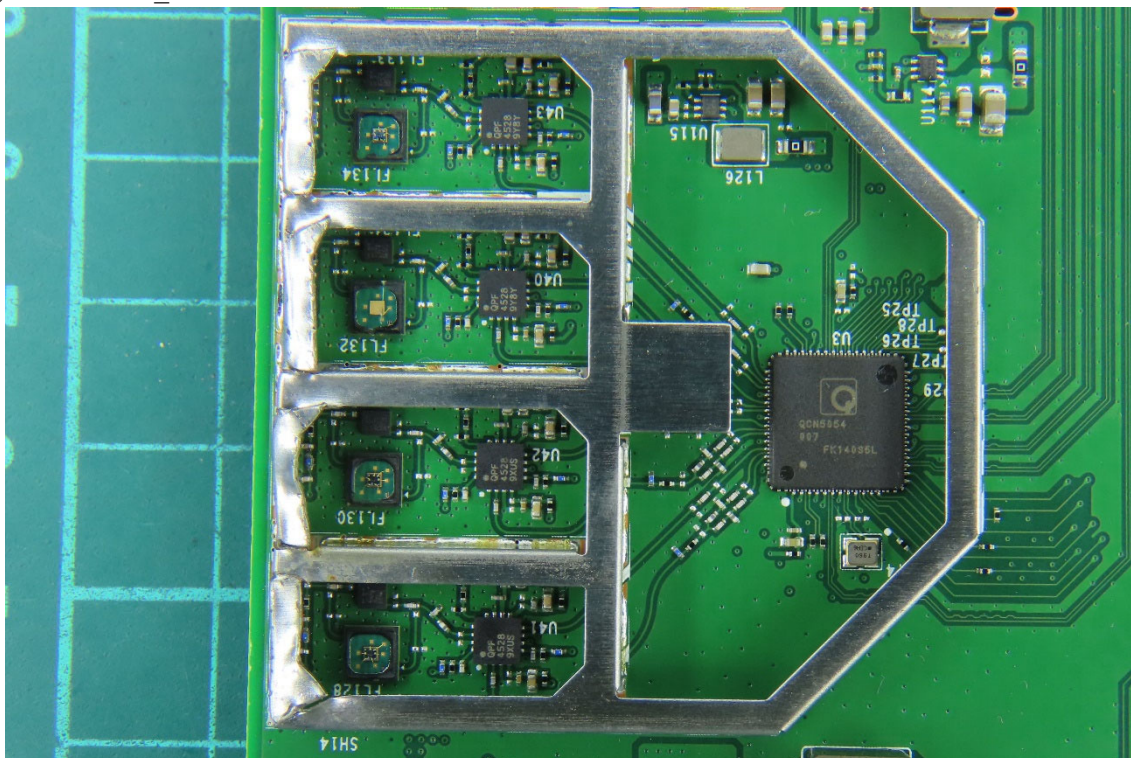
(11) EUT Photo_5GHz Module
