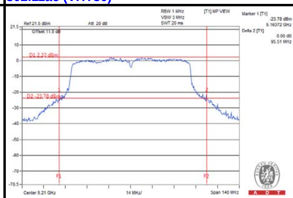
802.11ac (VHT80)
