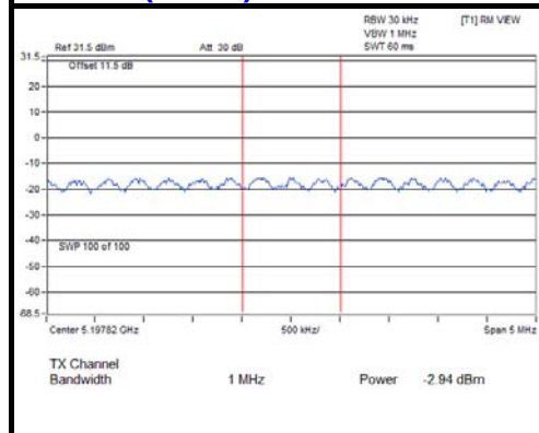
802.11ac (VHT40)
