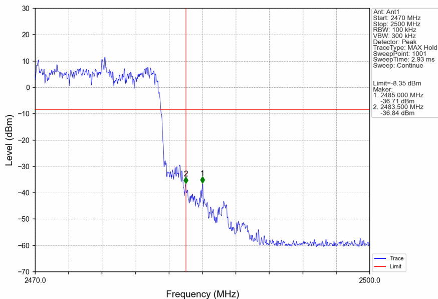
QHS 5M_HOPP_Ant1_NTNV
