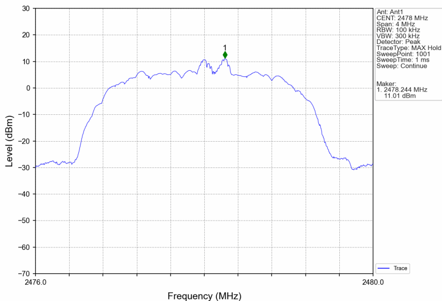
QHS 6M_HCH_2478MHz_Ant1_NTNV
