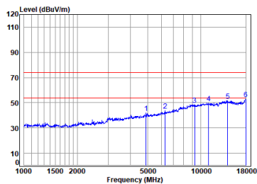
BLE_2M_TX_CH_38_Horizontal
