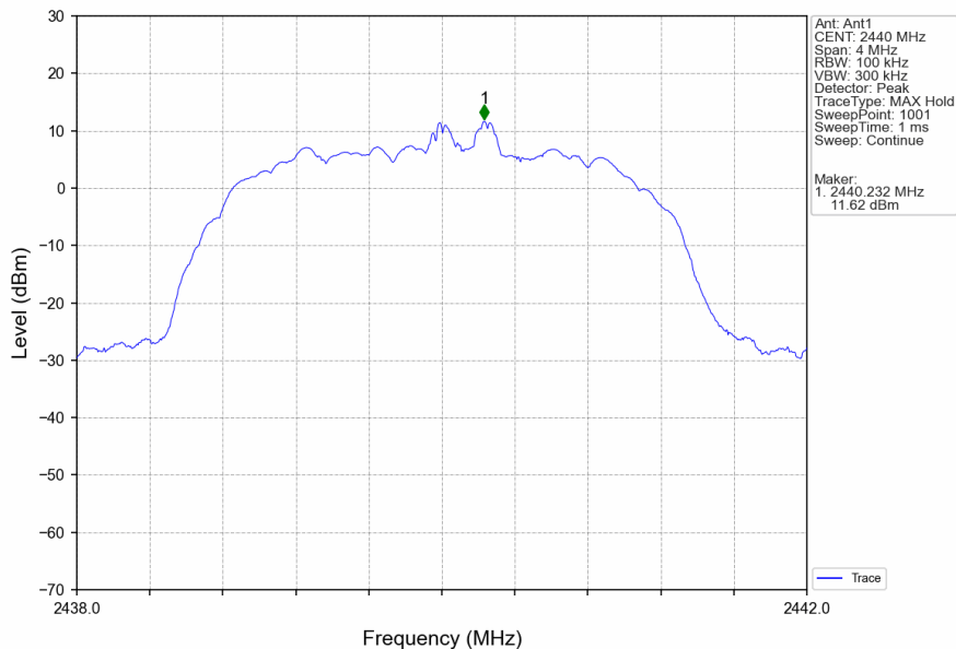
QHS 6M_MCH_2440MHz_Ant1_NTNV
