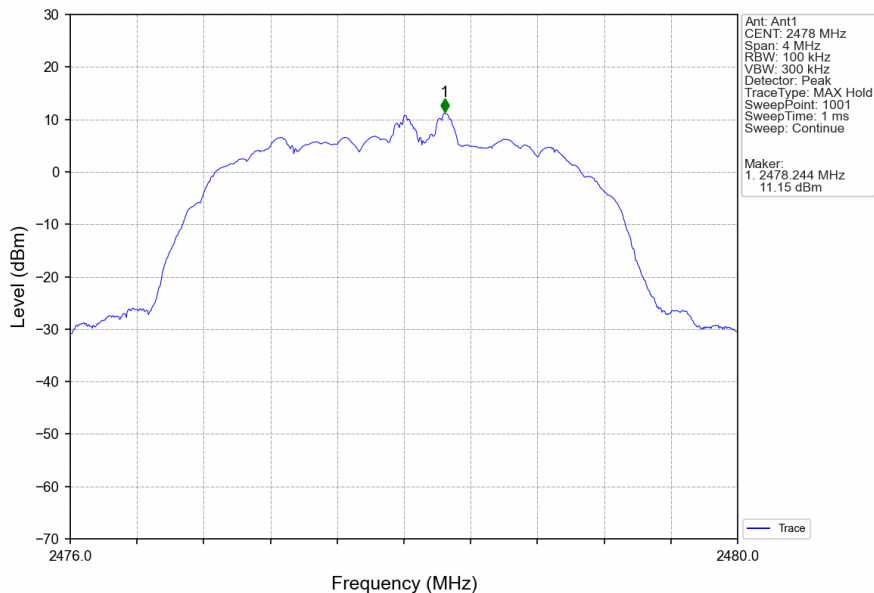
QHS 6M_HCH_2478MHz_Ant1_NTNV
