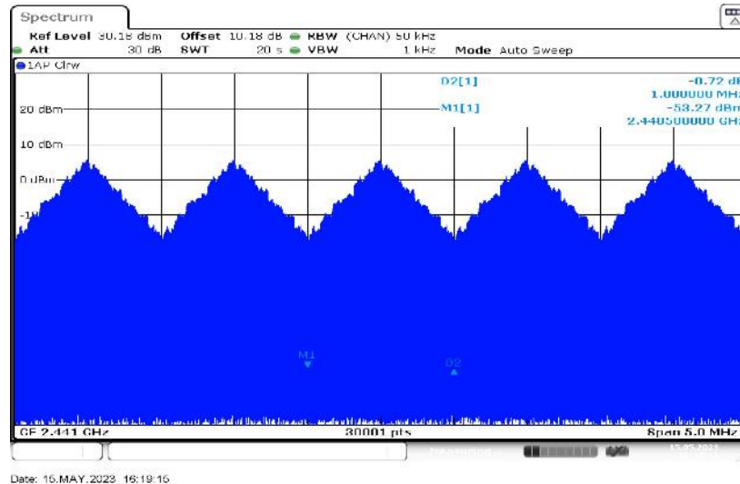
DH5 hopping
