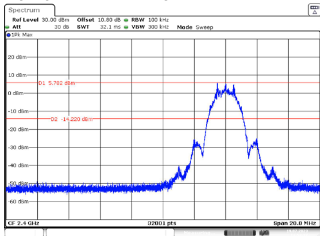
BLE 2M LOW CHANNEL BANDEDGE
