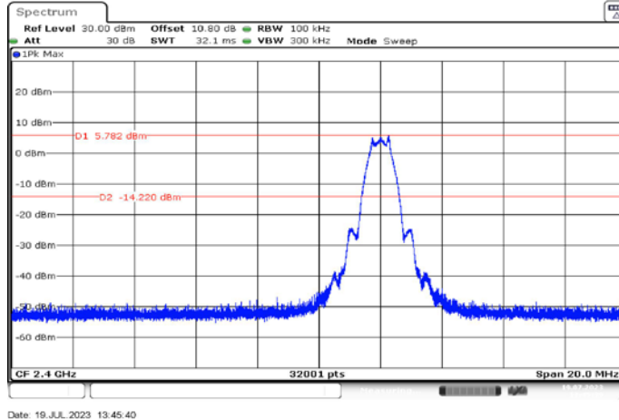
BLE 1M LOW CHANNEL BANDEDGE
