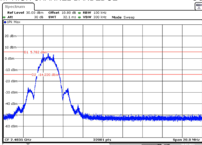
BLE 2M HIGH CHANNEL BANDEDGE
