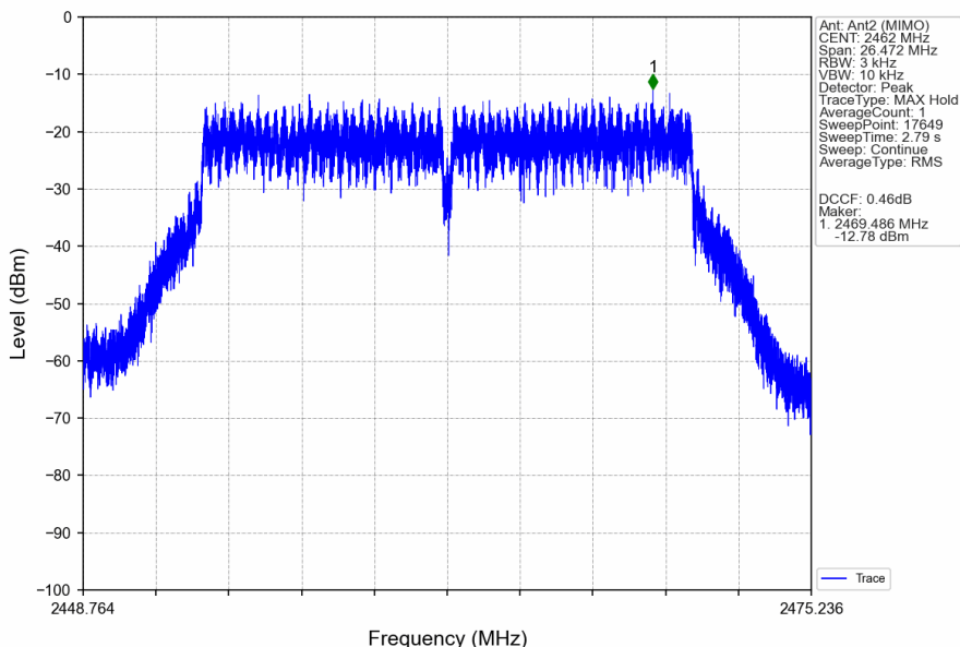
802.11n(HT20)_HCH_2462MHz_Ant2 (MIMO)_NTNV
