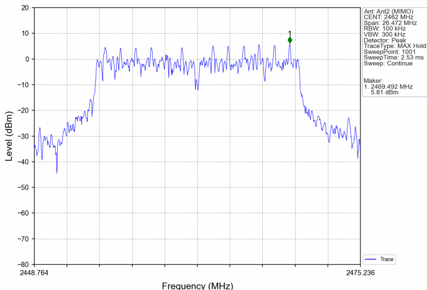
802.11n(HT20)_HCH_2462MHz_Ant2 (MIMO)_NTNV
