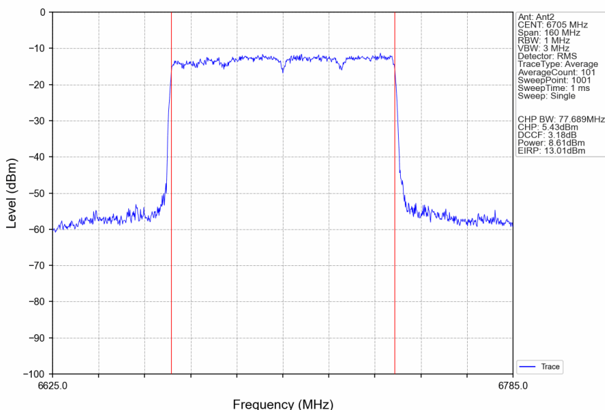
802.11ax(HEW80)_MCH_6705MHz_RU996_Left_Ant2_NTNV
