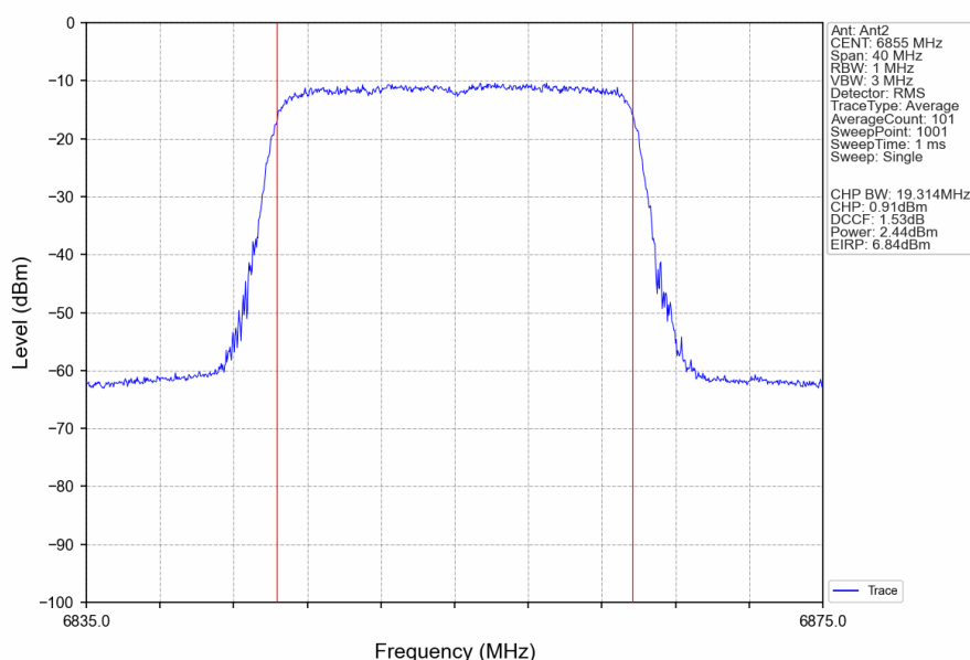
802.11ax(HEW20)_HCH_6855MHz_RU242_Left_Ant2_NTNV
