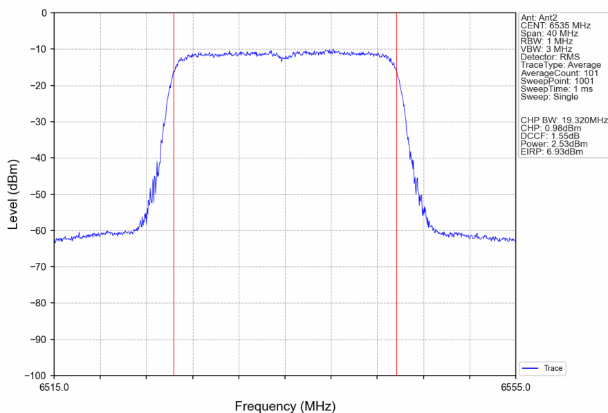
802.11ax(HEW20)_LCH_6535MHz_RU242_Left_Ant2_NTNV
