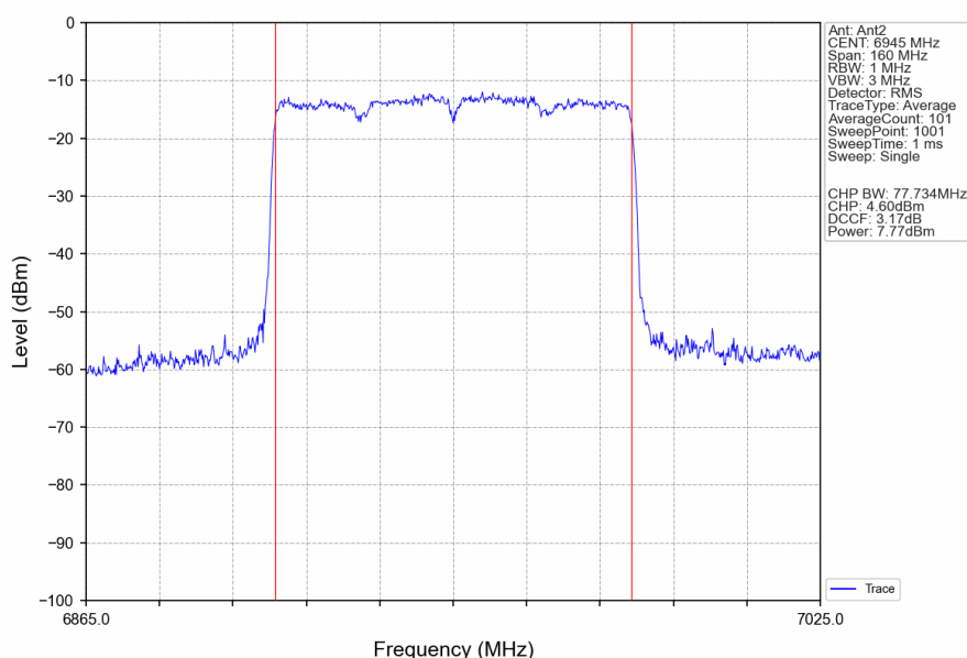
802.11ax(HEW80)_LCH_6945MHz_RU996_Left_Ant2_NTNV
