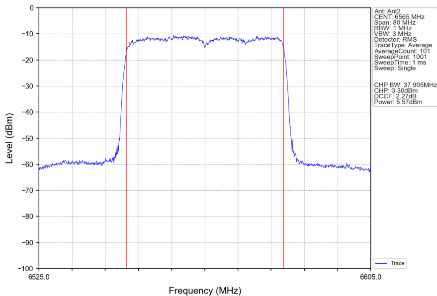
802.11ax(HEW40)_LCH_6565MHz_RU484_Left_Ant2_NTNV
