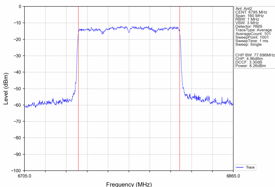
802.11ax(HEW80)_HCH_6785MHz_RU996_Left_Ant2_NTNV
