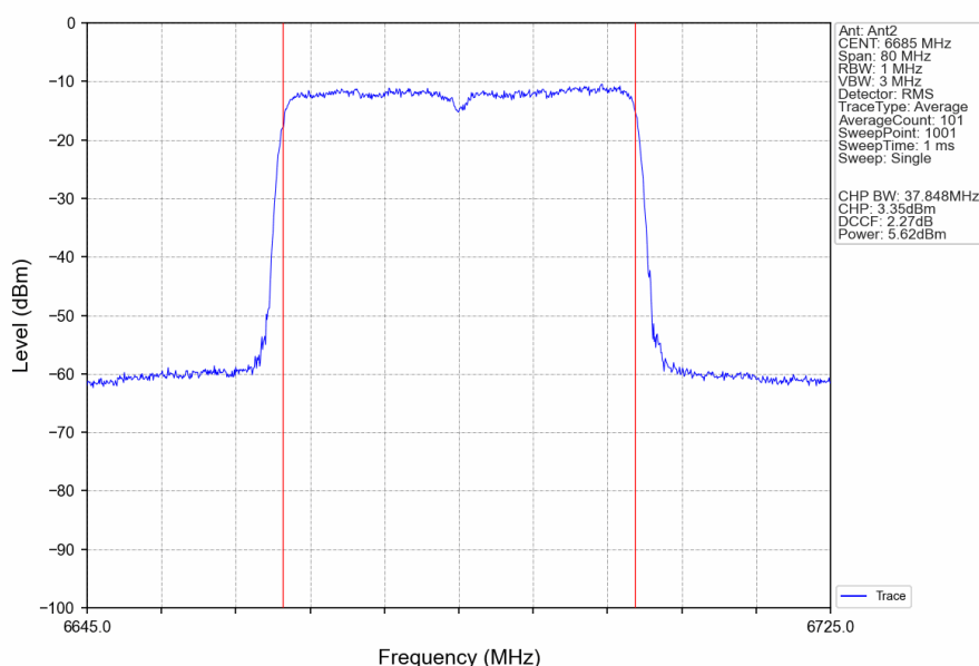
802.11ax(HEW40)_MCH_6685MHz_RU484_Left_Ant2_NTNV
