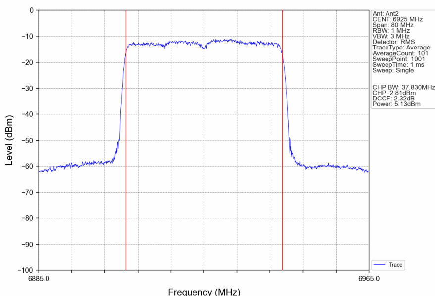
802.11ax(HEW40)_LCH_6925MHz_RU484_Left_Ant2_NTNV
