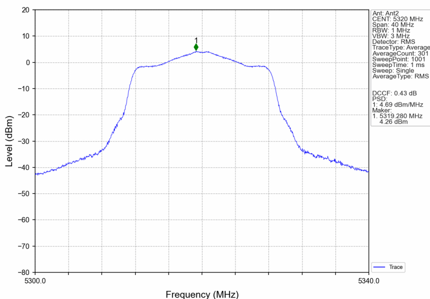
802.11a_HCH_5320MHz_MIMO_NTNV
