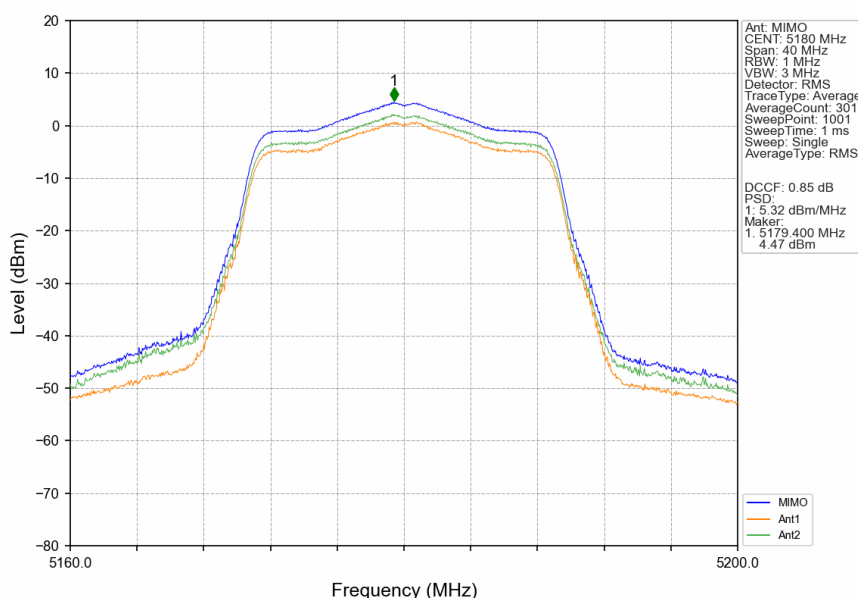
802.11n(HT20)_LCH_5180MHz_MIMO_NTNV
