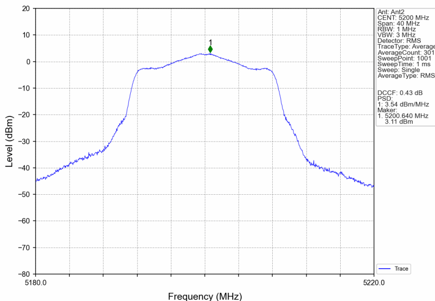
802.11a_MCH_5200MHz_MIMO_NTNV
