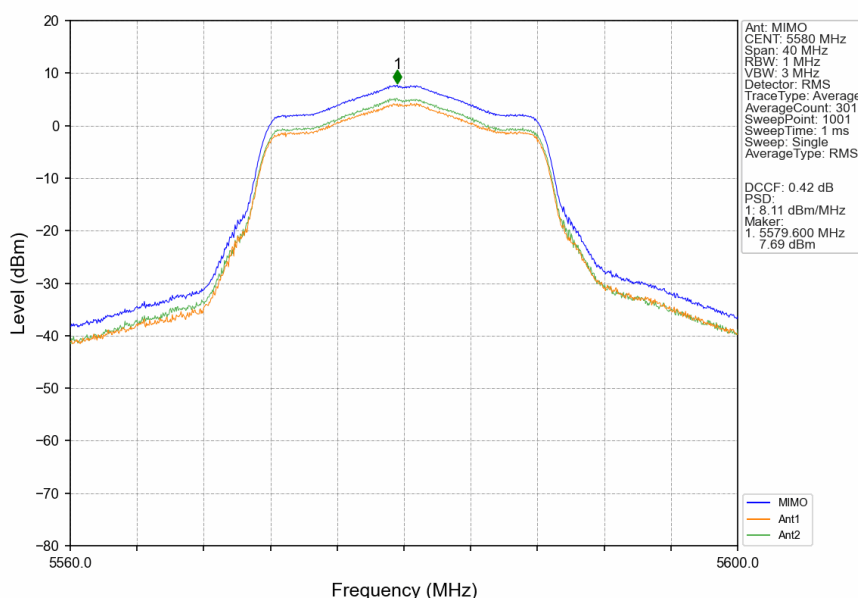
802.11a_MCH_5580MHz_MIMO_NTNV
