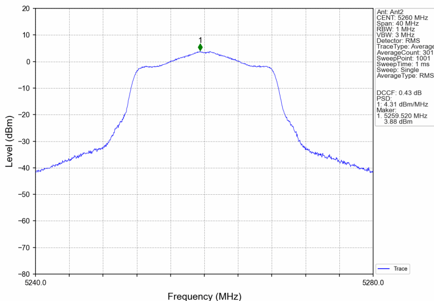
802.11a_LCH_5260MHz_MIMO_NTNV
