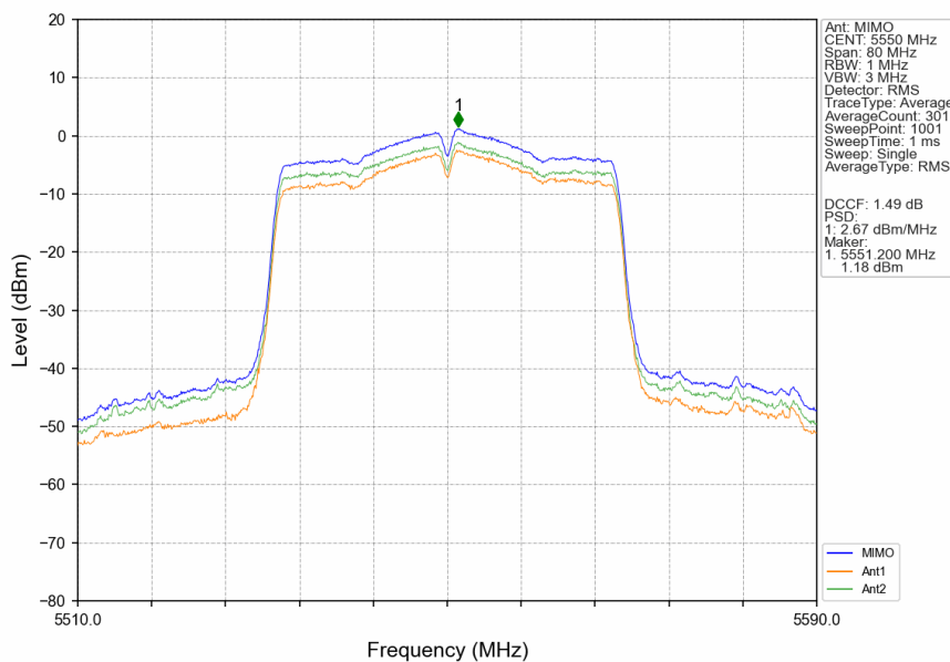
802.11n(HT40)_MCH_5550MHz_MIMO_NTNV
