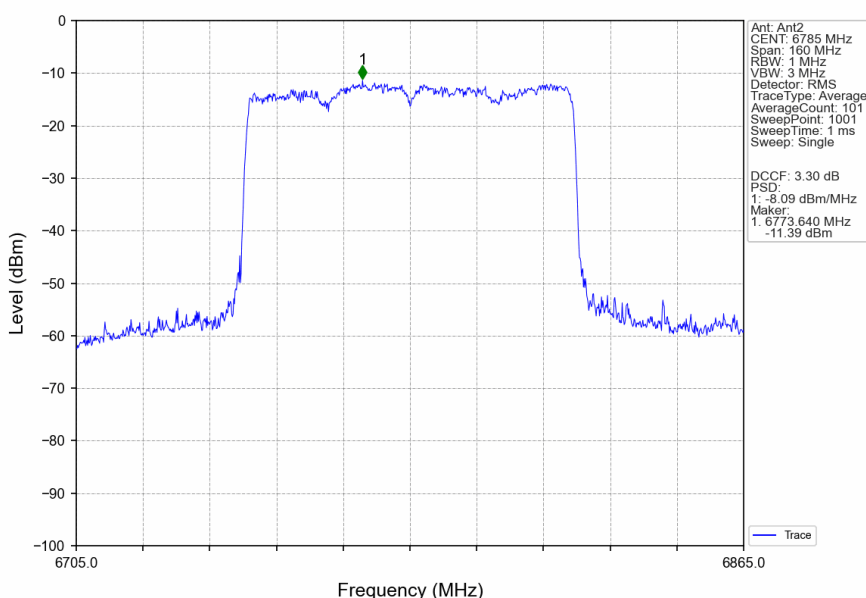
802.11ax(HEW80)_HCH_6785MHz_RU996_Left_Ant2_NTNV
