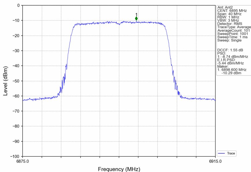
802.11ax(HEW20)_LCH_6895MHz_RU242_Left_Ant2_NTNV
