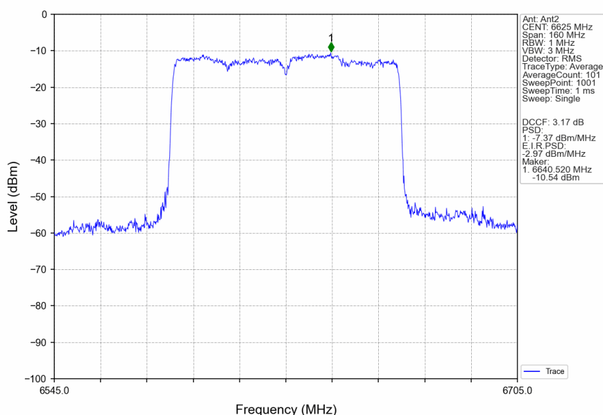
802.11ax(HEW80)_LCH_6625MHz_RU996_Left_Ant2_NTNV
