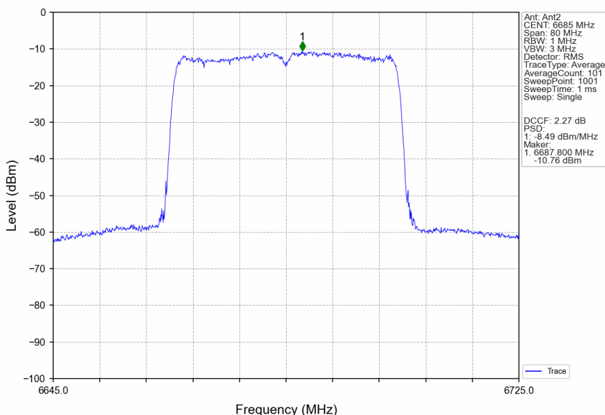
802.11ax(HEW40)_MCH_6685MHz_RU484_Left_Ant2_NTNV
