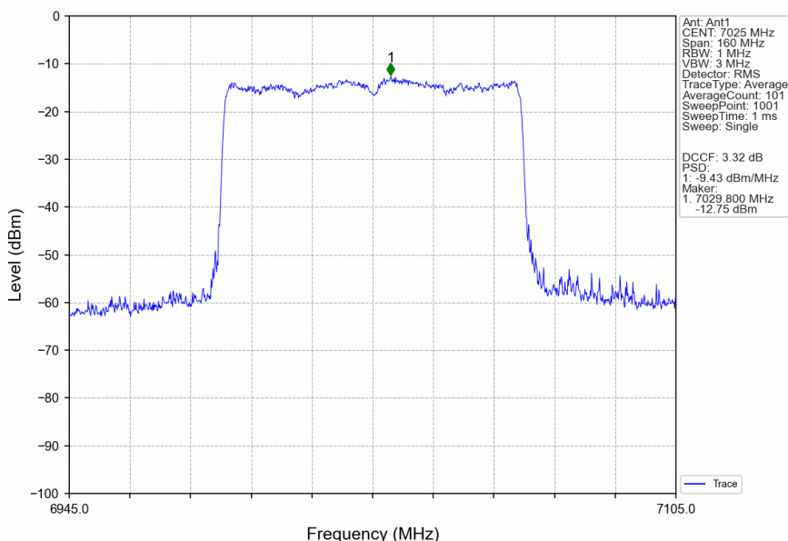
802.11ax(HEW80)_HCH_7025MHz_RU996_Left_Ant1_NTNV
