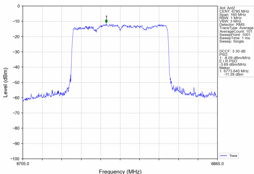
802.11ax(HEW80)_HCH_6785MHz_RU996_Left_Ant2_NTNV
