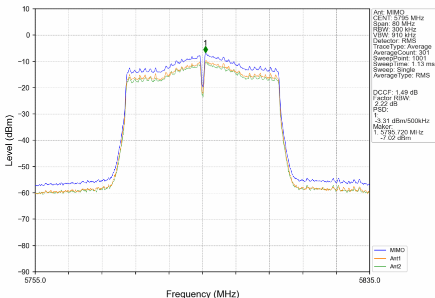
802.11n(HT40)_HCH_5795MHz_MIMO_NTNV
