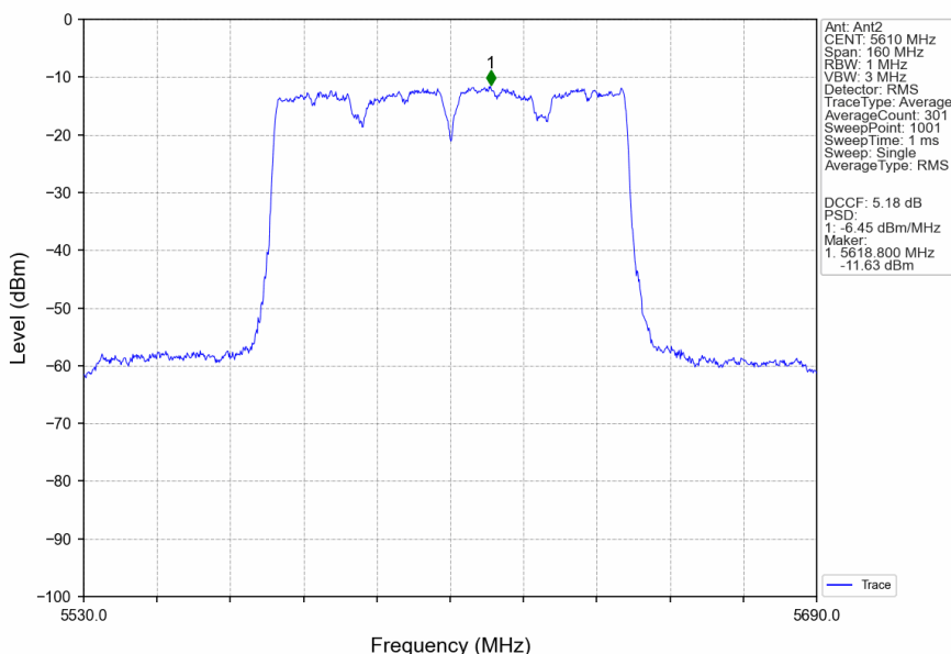
802.11ac(VHT80)_HCH_5610MHz_Ant2_NTNV
