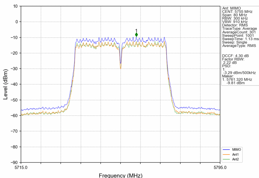
802.11ac(VHT40)_LCH_5755MHz_MIMO_NTNV
