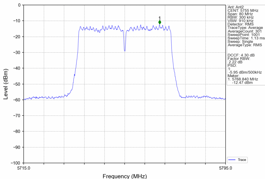
802.11ac(VHT40)_LCH_5755MHz_MIMO_NTNV
