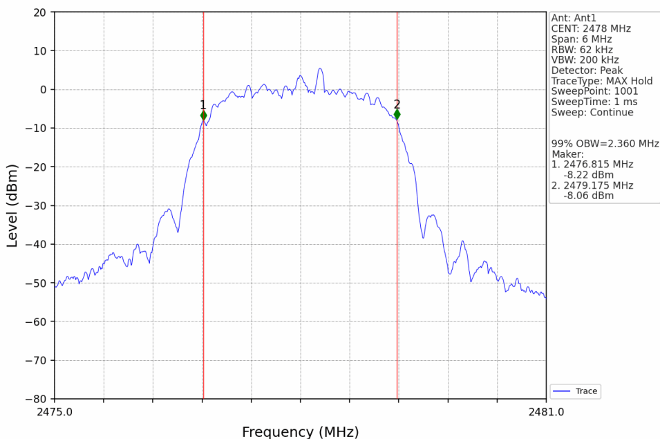
QHS2_HCH_2478MHz_Ant1_NTNV
