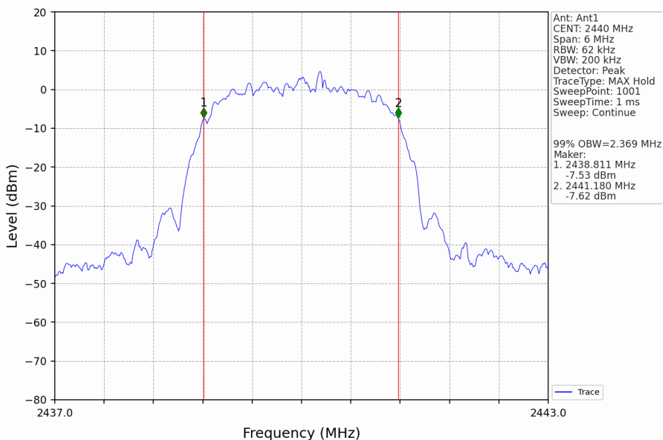
QHS4_MCH_2440MHz_Ant1_NTNV
