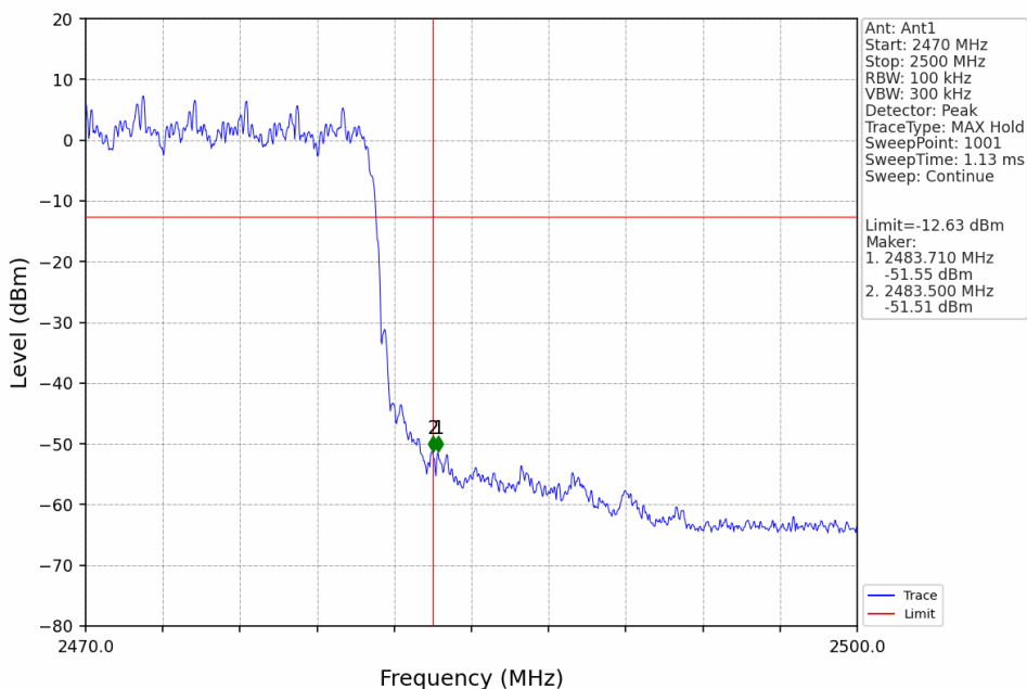
QHS2_HOPP_Ant1_NTNV
