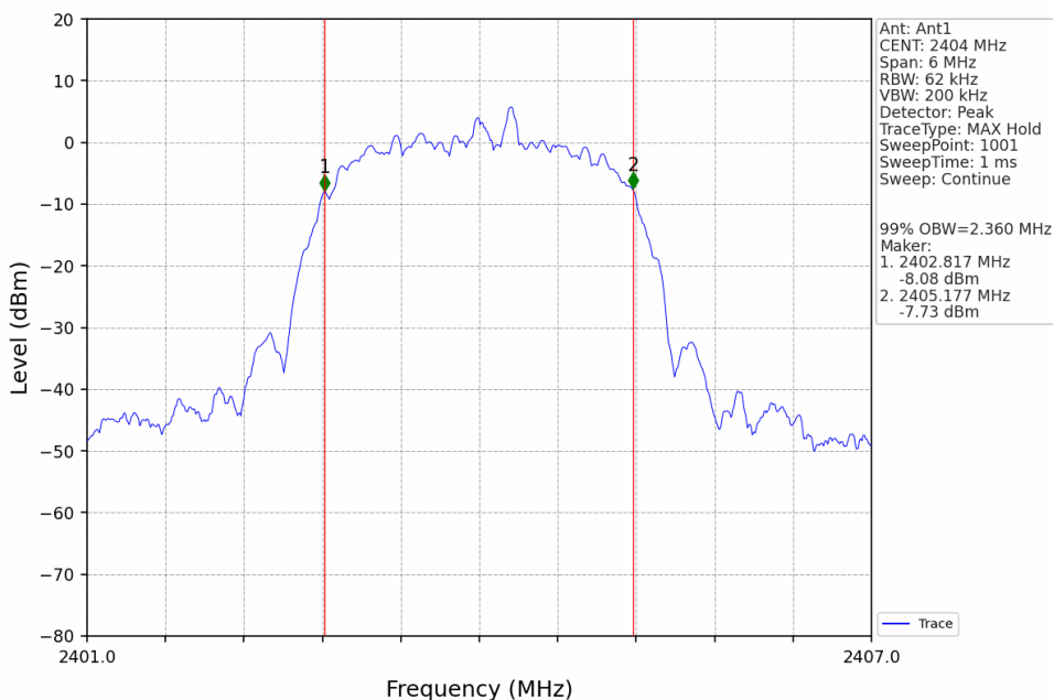
QHS2_LCH_2404MHz_Ant1_NTNV
