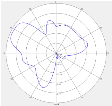
5500MHZ H-pol
