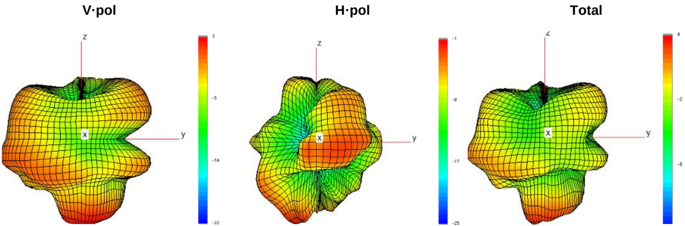
2450MHZ 3D
