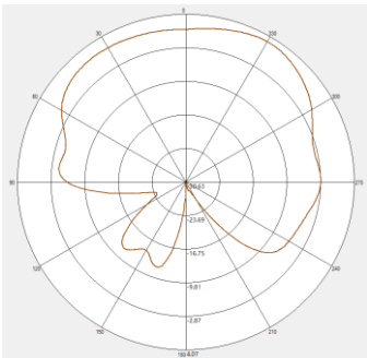
2400MHZ H-pol
