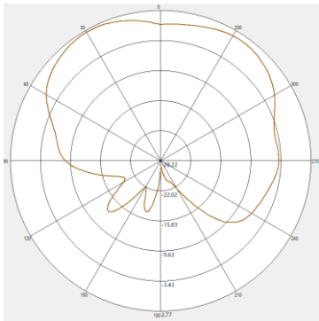
2500MHZ H-pol
