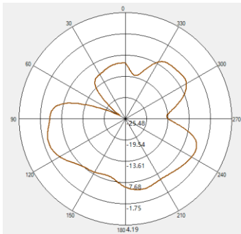
2450MHZ V-pol
