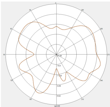
2400MHZ H-pol
