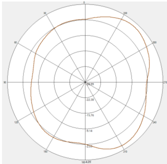
2400MHZ V-pol
