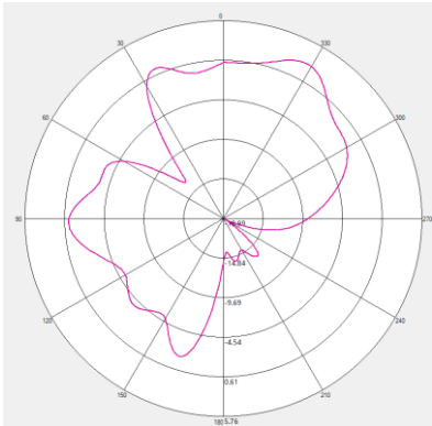
6550MHZ H-pol
