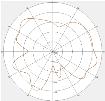
2450MHZ H-pol
