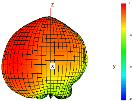
H-Pol
