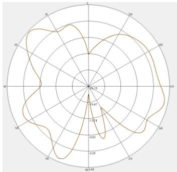
2500MHZ H-pol
