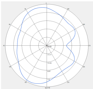
5150MHZ V-pol
