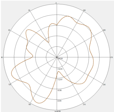
2450MHZ H-pol
