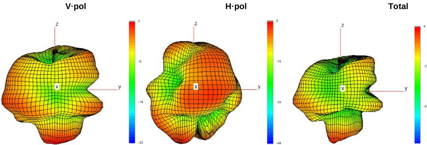
2450MHZ 3D
