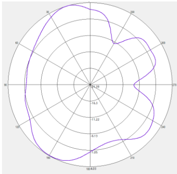
5850MHZ V-pol
