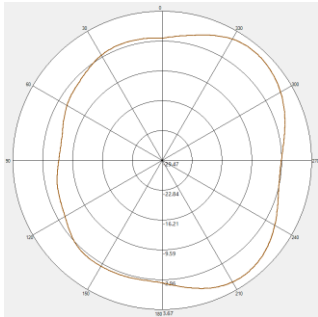
2450MHZ V-pol
