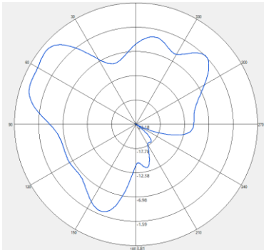
5150MHZ H-pol
