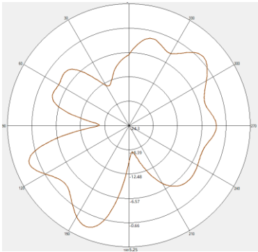
2400MHZ H-pol
