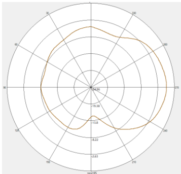
2500MHZ V-pol
