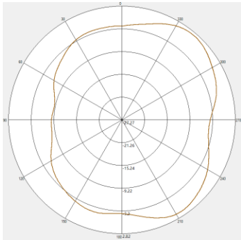
2500MHZ V-pol
