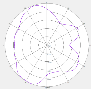
5950MHZ V-pol
