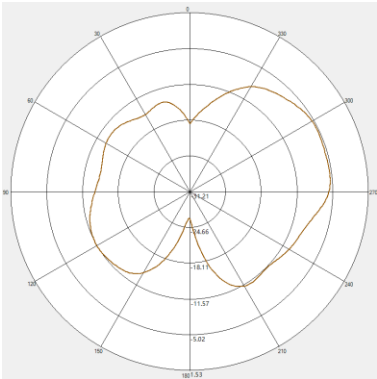
2500MHZ V-pol
