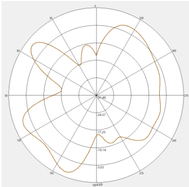
2500MHZ H-pol
