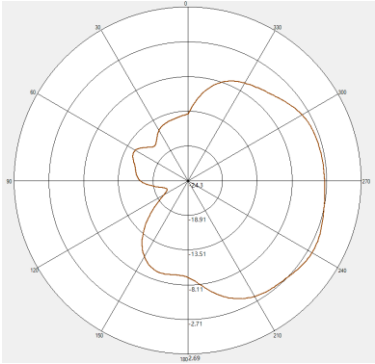
2400MHZ V-pol
