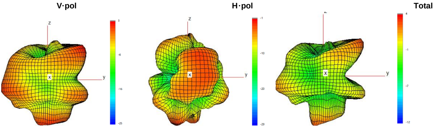
2500MHZ 3D
