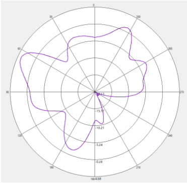
5950MHZ H-pol
