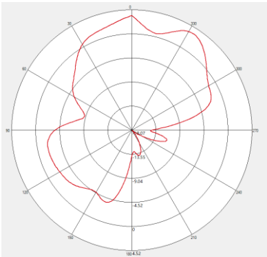
7120MHZ H-pol
