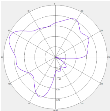
5850MHZ H-pol
