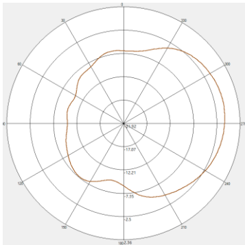
2400MHZ V-pol
