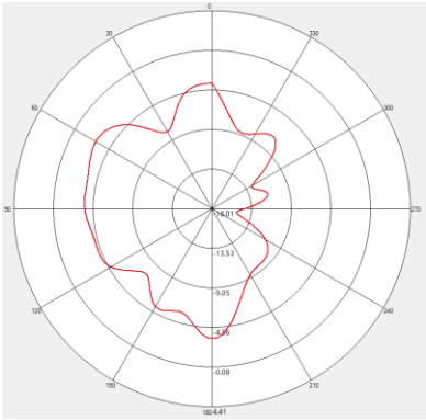
7120MHZ V-pol
