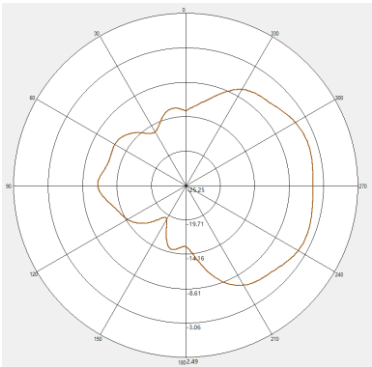
2450MHZ V-pol
