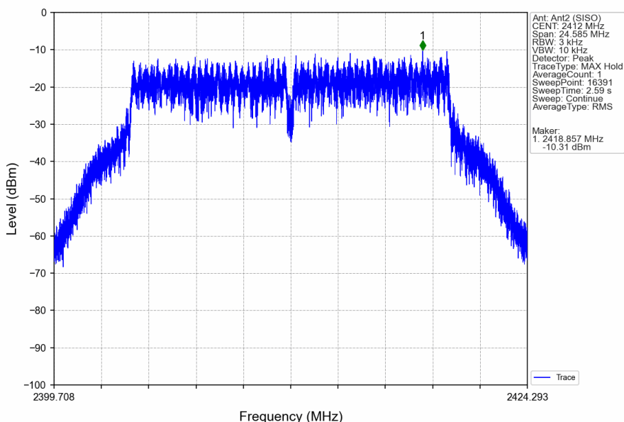
802.11g_LCH_2412MHz_Ant2 (SISO)_NTNV
